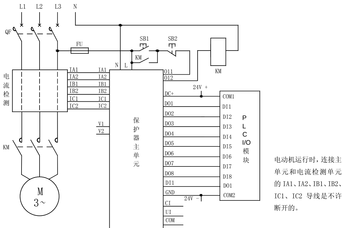
AMDG-□/D7 系列电动机保护器应用电气原理图
