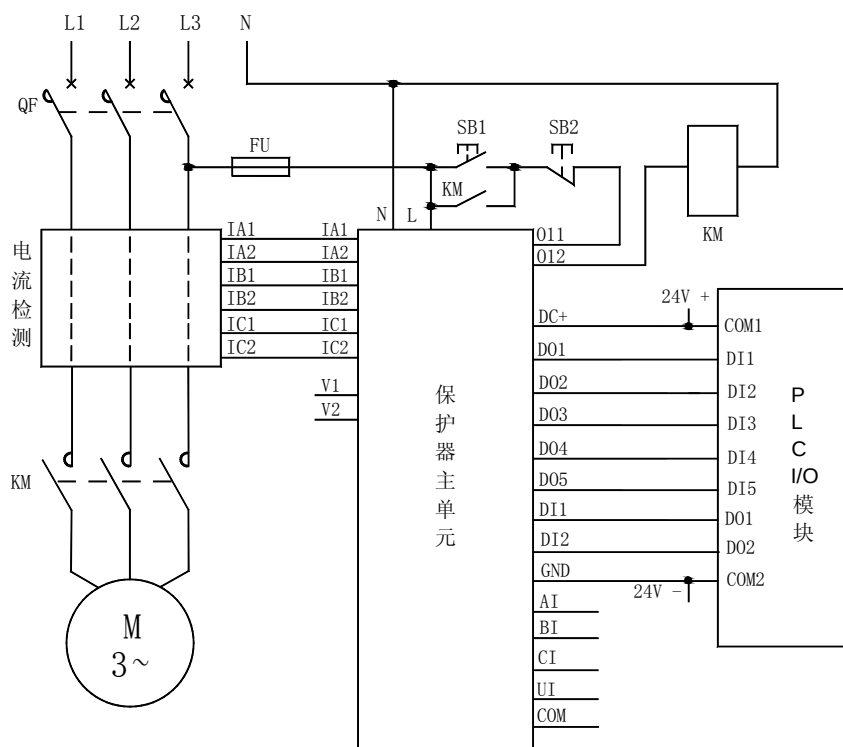
AMDG-□/D8 系列电动机保护器应用电气原理图
