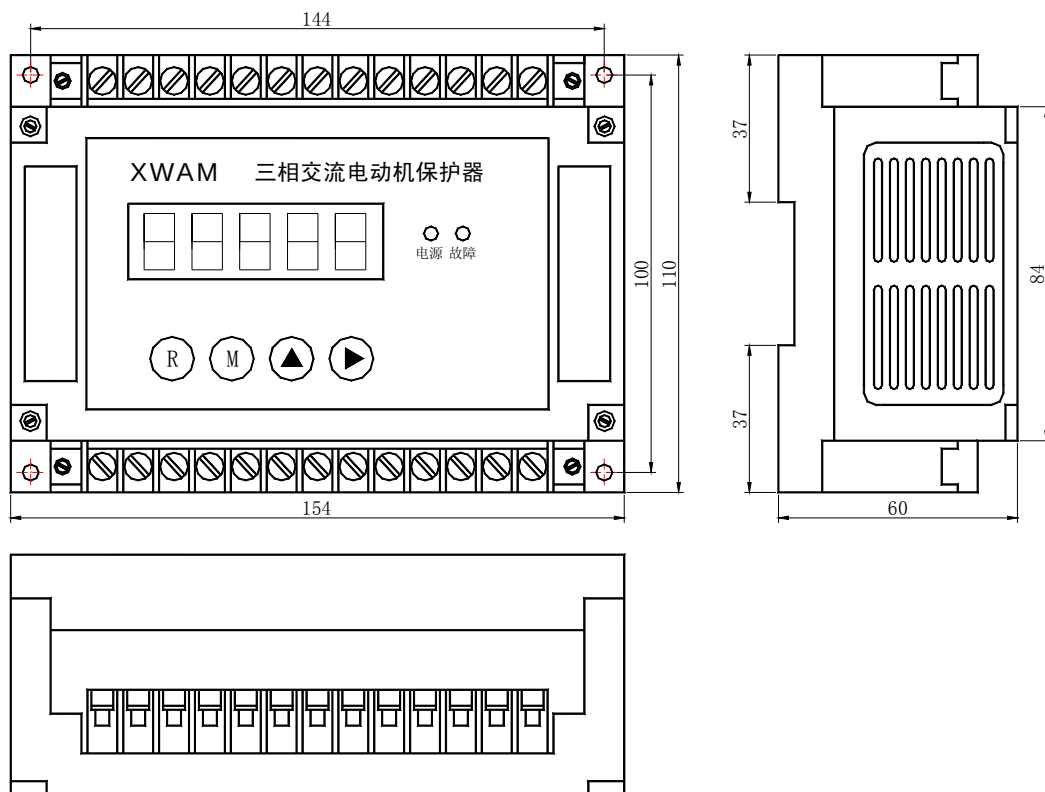
AMDG-X/E1 系列电动机保护器主单元外形及安装孔尺寸
