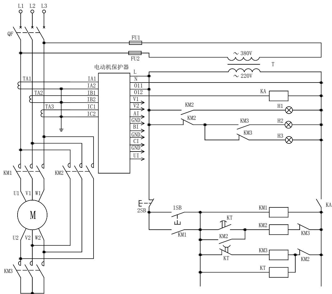
图 2 电动机保护器用于星/三角起动（检测线电流）电气原理图
