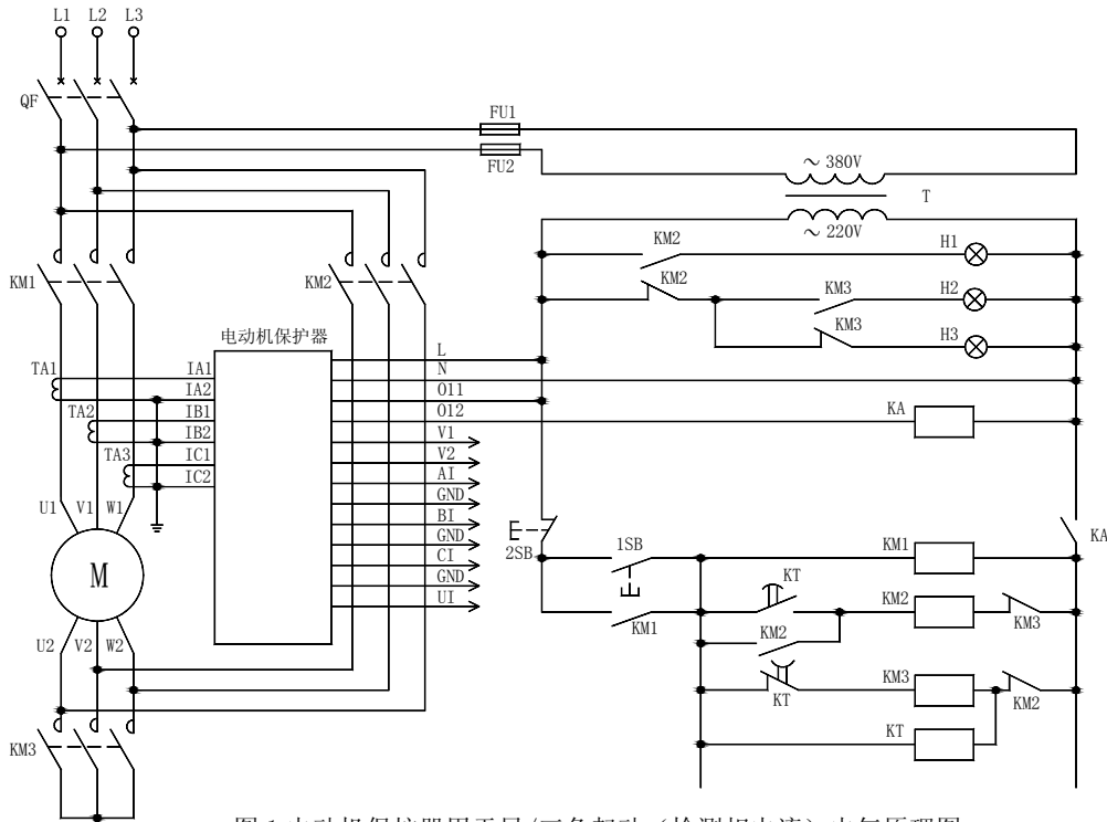
图 1 电动机保护器用于星/三角起动（检测相电流）电气原理图
