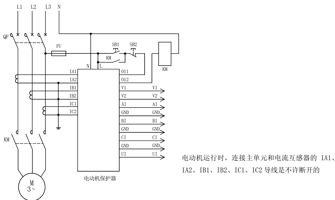
AMDG-X/F1 系列电动机保护器应用电气原理图
