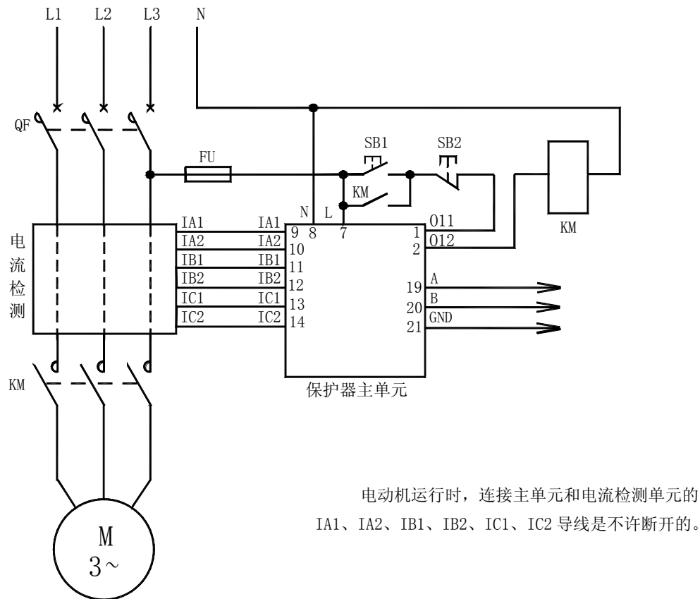
AMDP-□/C3 系列电动机保护器应用电气原理图
