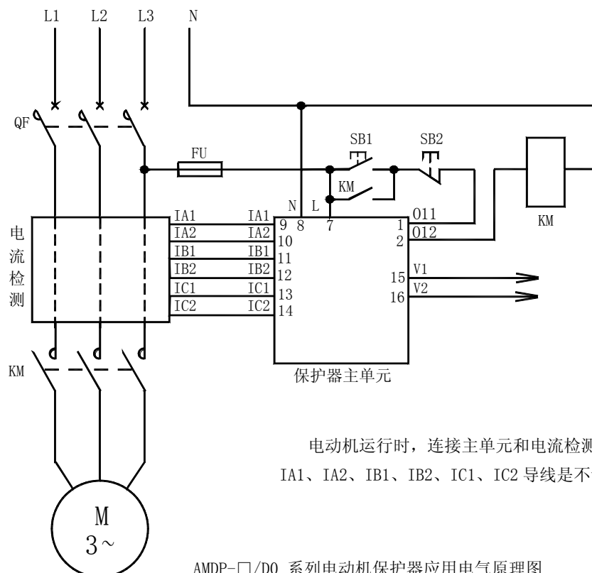
AMDP-□/D0 系列电动机保护器应用电气原理图
