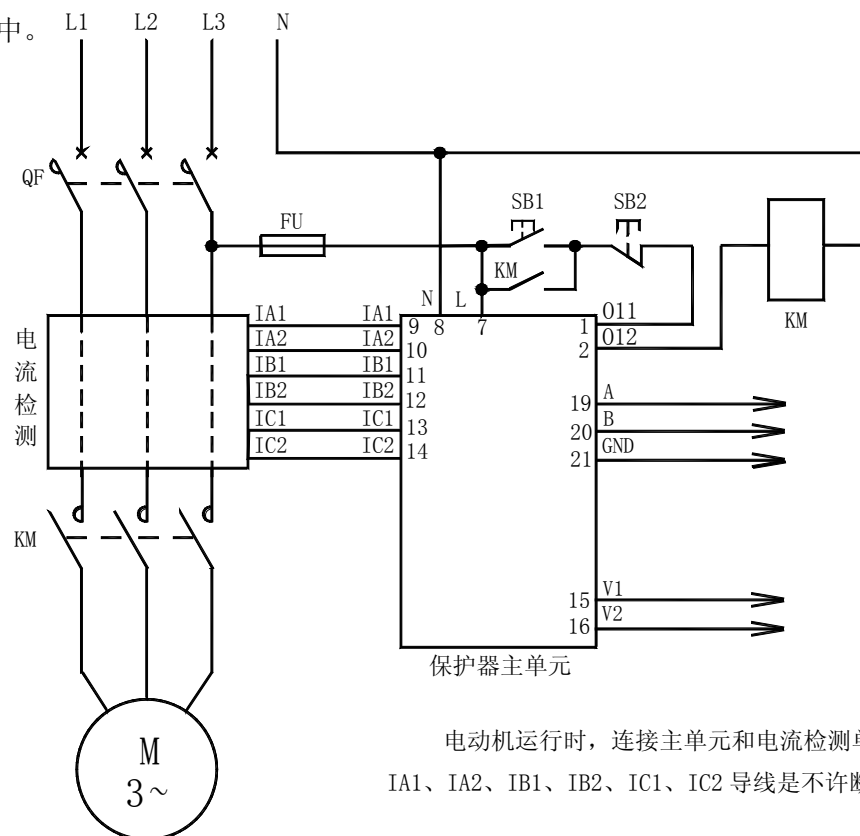
AMDP-□/D3 系列电动机保护器应用电气原理图
