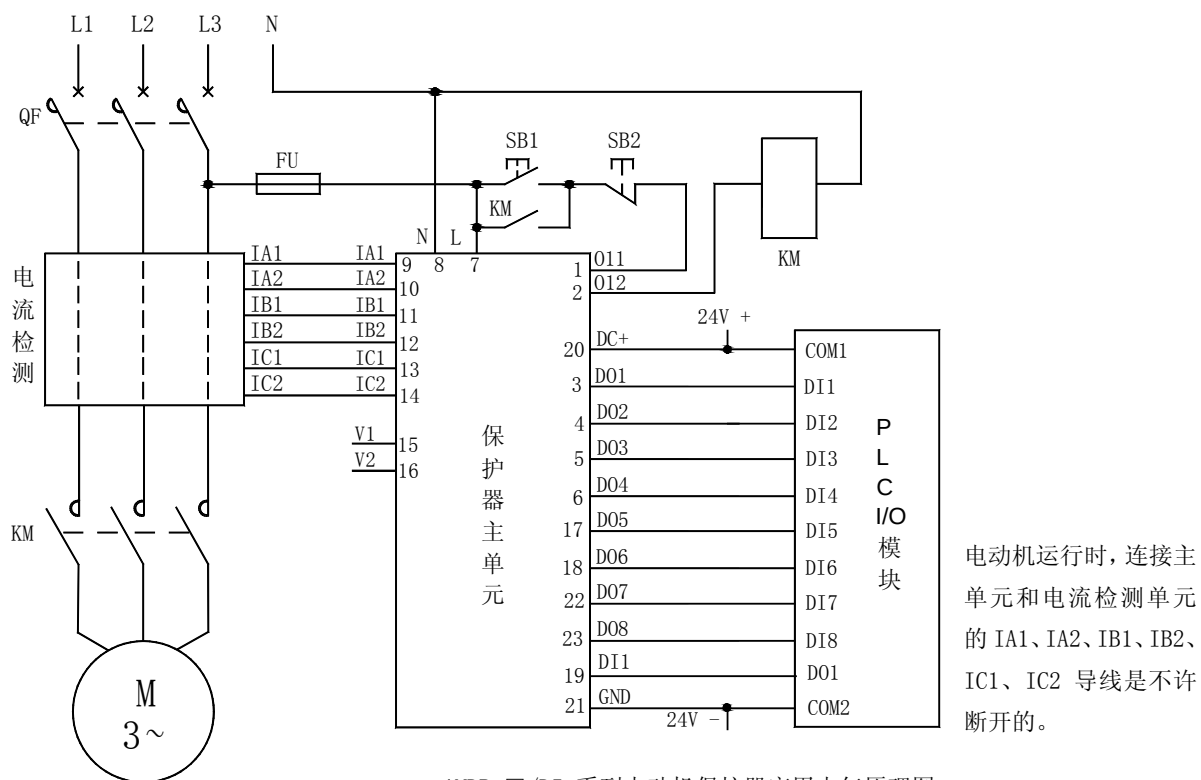
AMDP-□/D5 系列电动机保护器应用电气原理图
