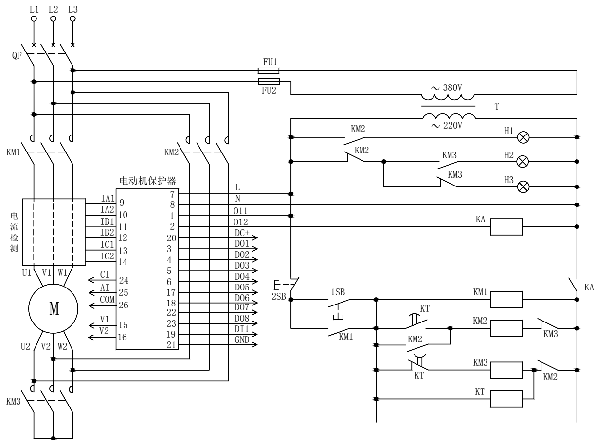
图 2 电动机保护器用于星/三角启动（检测线电流）电气原理图
