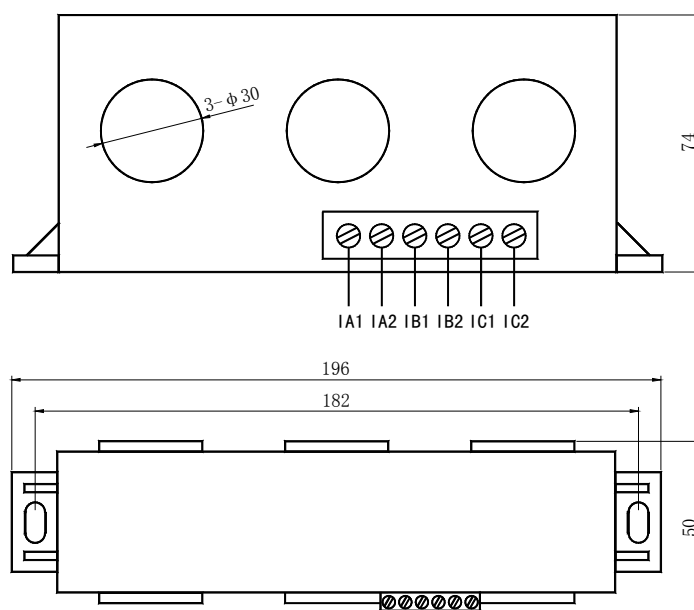
穿线孔直径 Φ30mm 的电流检测单元外形及安装尺寸
