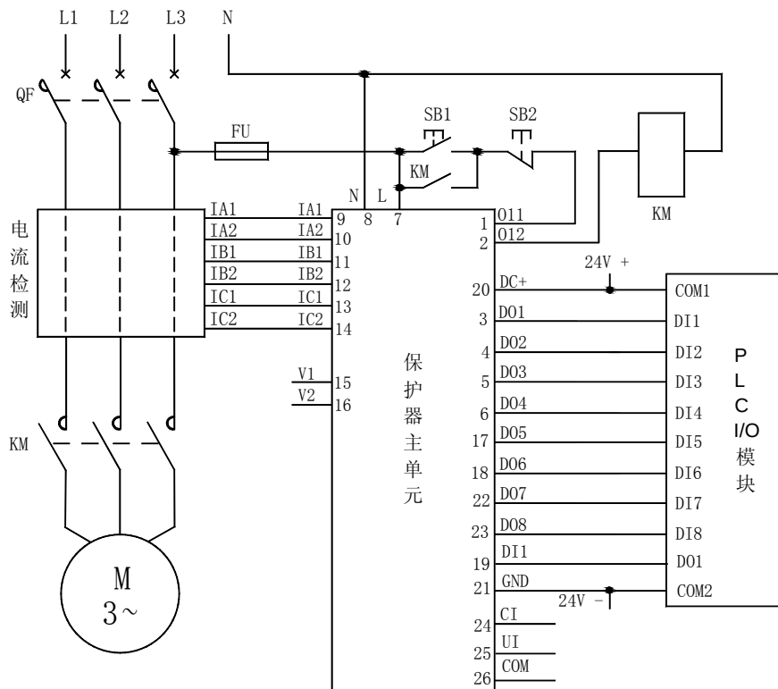
AMDP-□/D7 系列电动机保护器应用电气原理图
