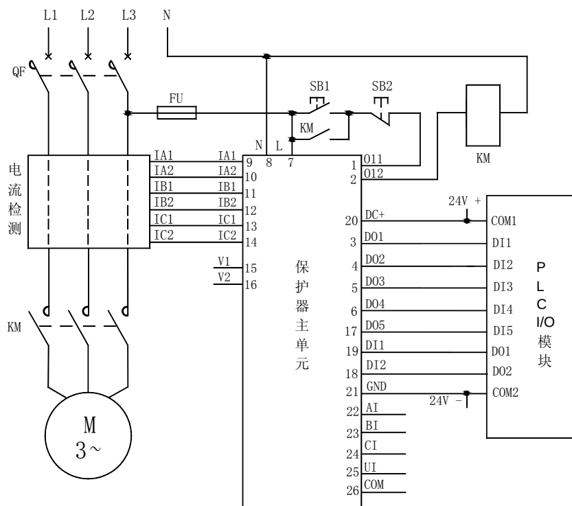
AMDP-□/D8 系列电动机保护器应用电气原理图
