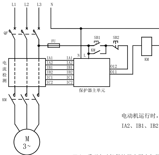
AMDS-□/A 系列电动机保护器应用电气原理图
