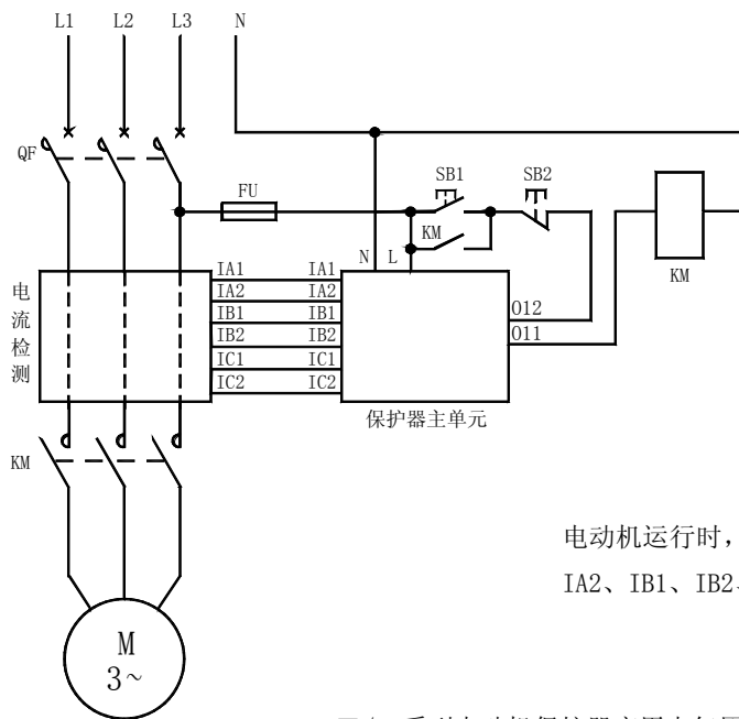
AMDS-□/B 系列电动机保护器应用电气原理图
