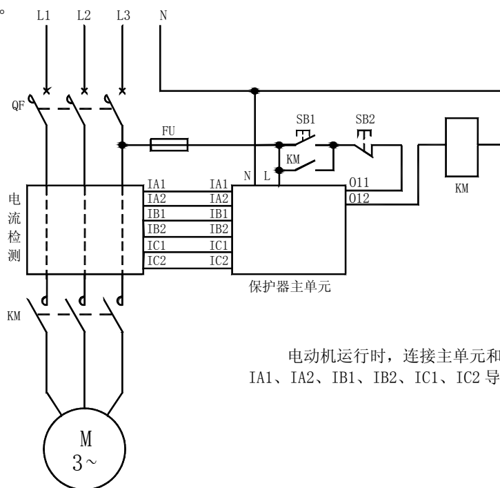
AMDS-□/C 系列电动机保护器应用电气原理图
