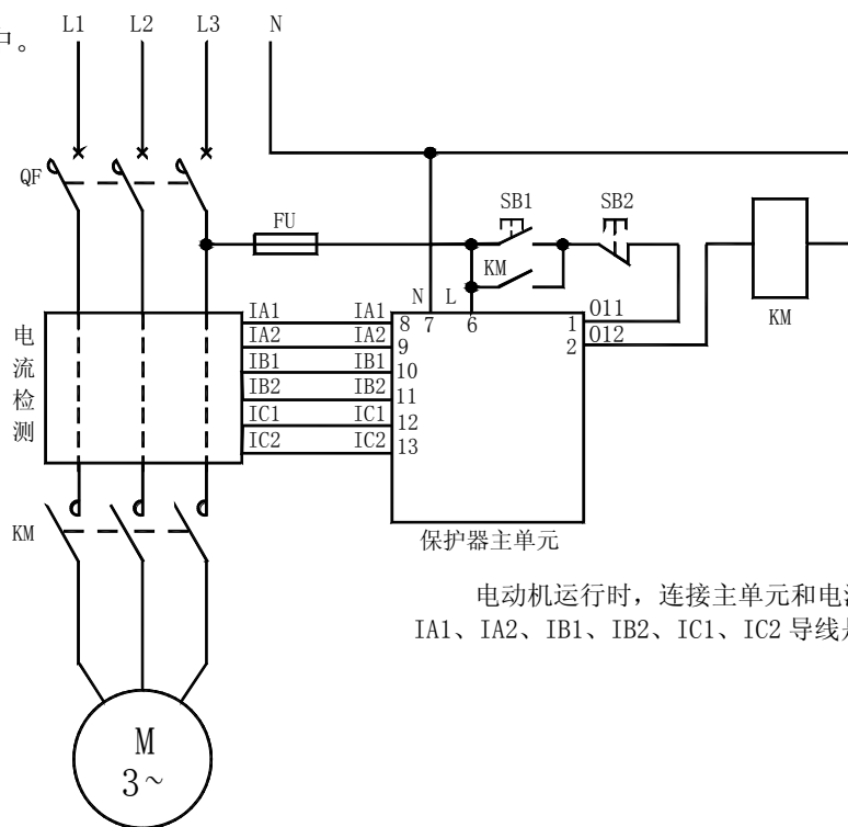
AMDT-□/C 系列电动机保护器应用电气原理图
