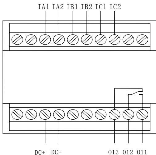
AMDG-□/A001 系列保护器主单元端子图
