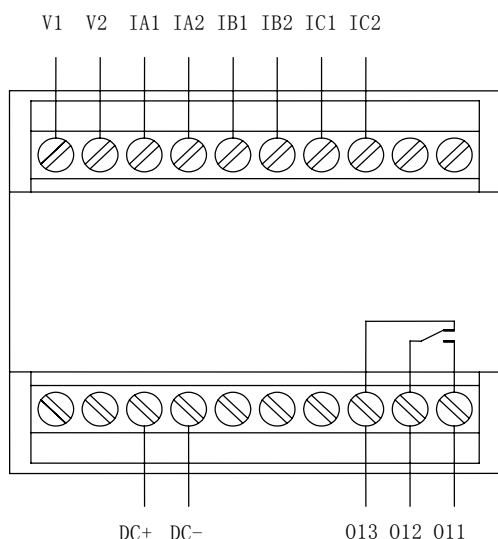
AMDG-□/A031 系列保护器主单元端子图
