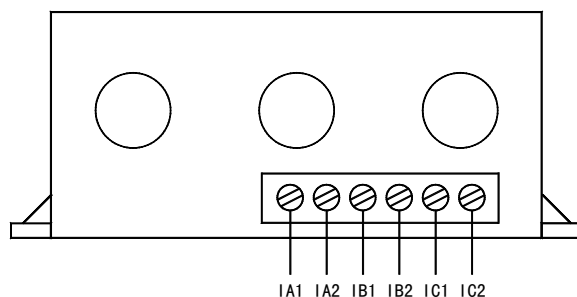
AMDG-□/A0□□ 系列电动机保护器电流检测单元接线端子图
