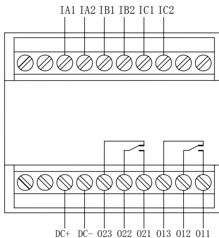
AMDG-□/A002 系列保护器主单元端子图
