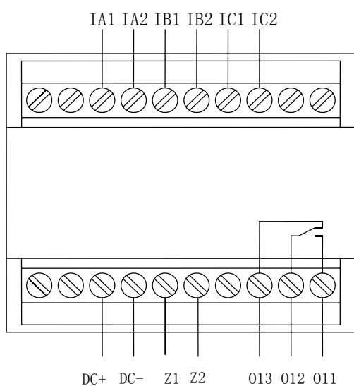
AMDG-□/A011 系列保护器主单元端子图
