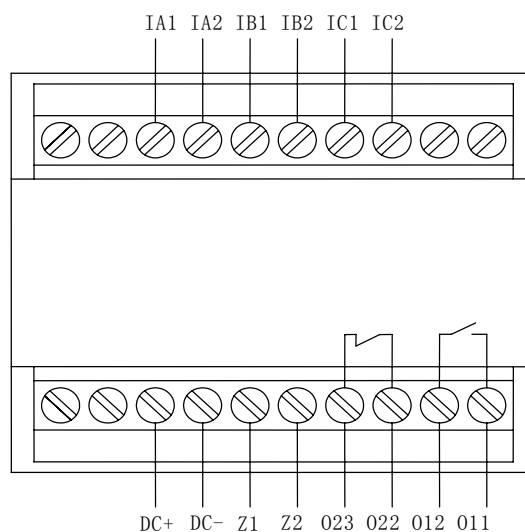
AMDG-□/A014 系列保护器主单元端子图
