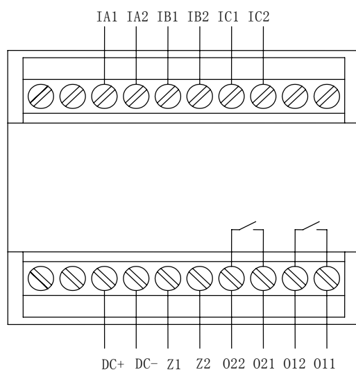
AMDG-□/A013 系列保护器主单元端子图
