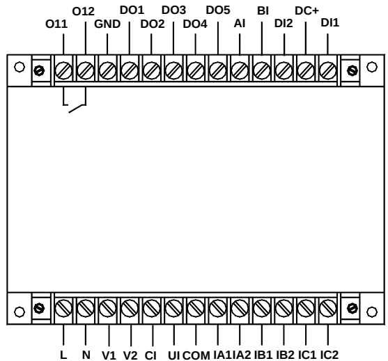
AMDG-X/F8□1 系列保护器主单元接线端子图
