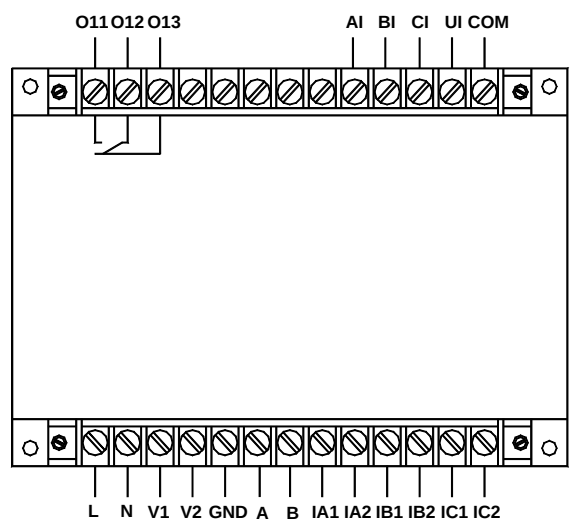
AMDG-X/F4□1 系列保护器主单元端子图
