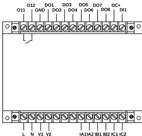
AMDG-X/F5□1 系列保护器主单元接线端子图
