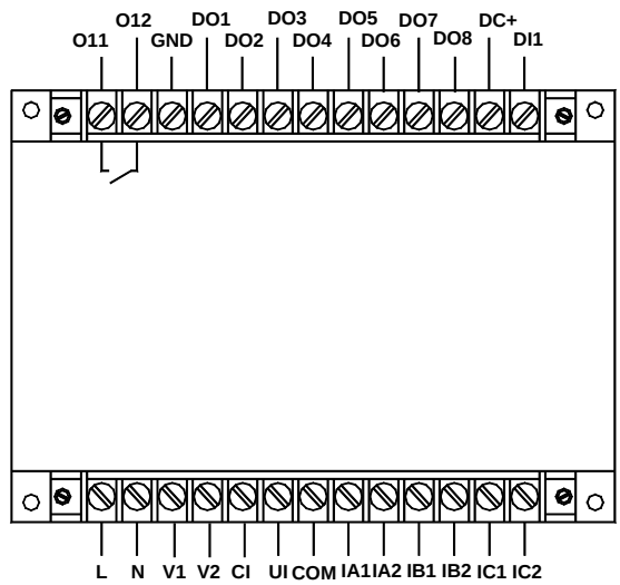
AMDG-X/F7□1 系列保护器主单元接线端子图
