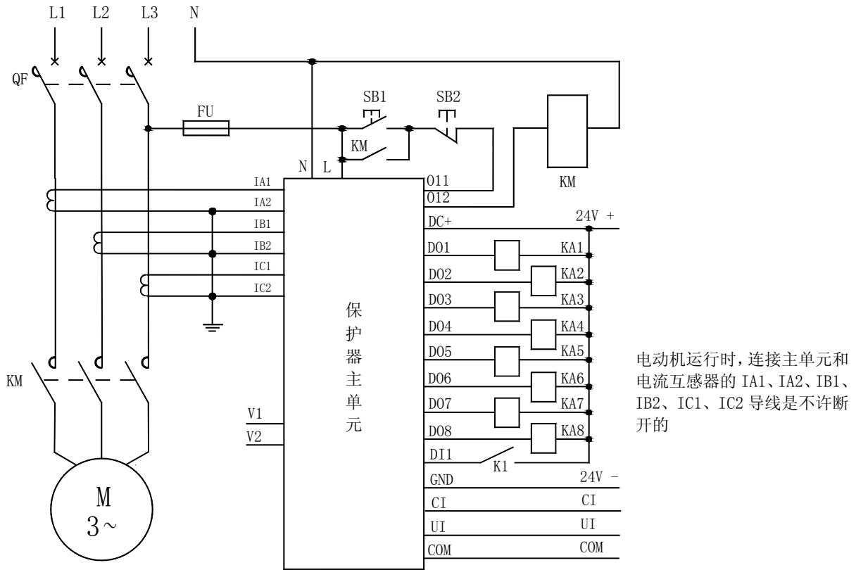
AMDG-X/F7□1 系列电动机保护器 DO 连接继电器电气原理图
