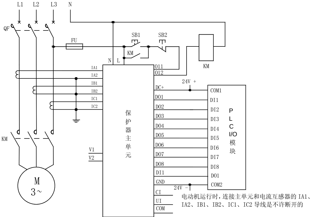
AMDG-X/F7□1 系列电动机保护器 DO 连接 PLC 电气原理图
