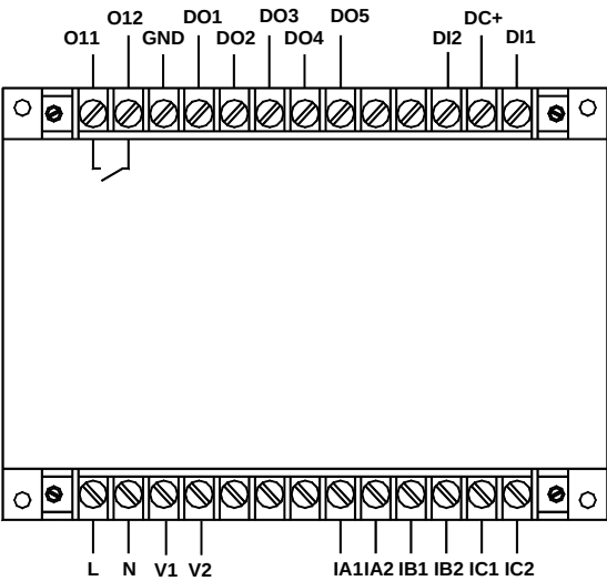
AMDG-X/F6□1 系列保护器主单元接线端子图
