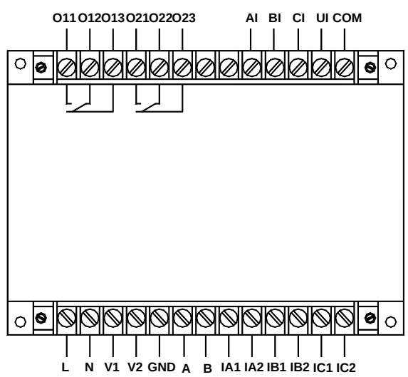
AMDG-X/F4□2 系列保护器主单元端子图
