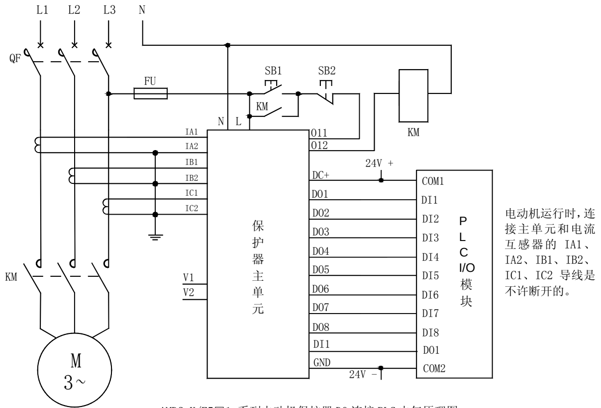
AMDG-X/F5□1 系列电动机保护器 DO 连接 PLC 电气原理图
