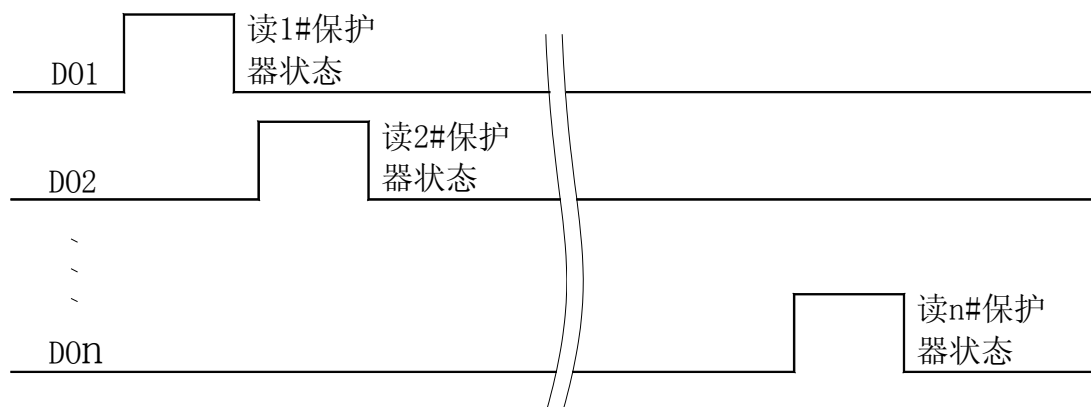
PLC 读取多台 AMDG-X/F6、AMDG-X/F8 系列电动机保护器时序图
