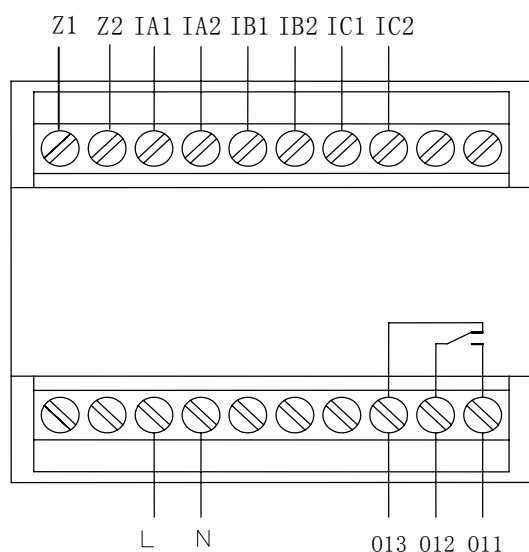
AMDS-□/A011 系列保护器主单元端子图
