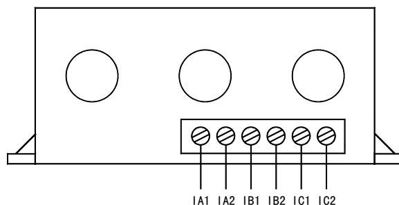
AMDS-□/A0□□ 系列电动机保护器电流检测单元接线端子图
