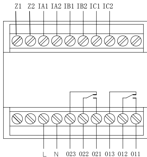
AMDS-□/A012 系列保护器主单元端子图
