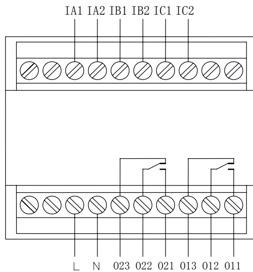
AMDS-□/A002 系列保护器主单元端子图
