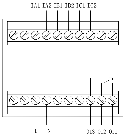
AMDS-□/A001 系列保护器主单元端子图
