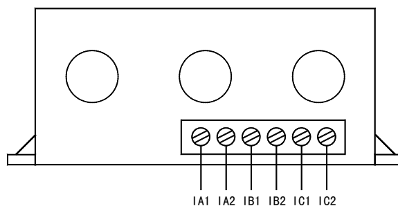
AMDS-□/B 系列电动机保护器电流检测单元接线端子图
