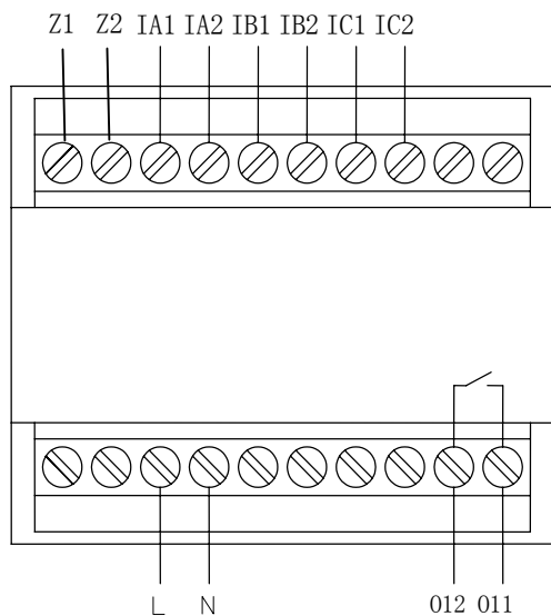
AMDS-□/B011 系列保护器主单元端子图
