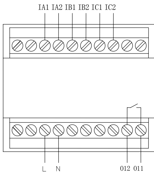
AMDS-□/B001 系列保护器主单元端子图
