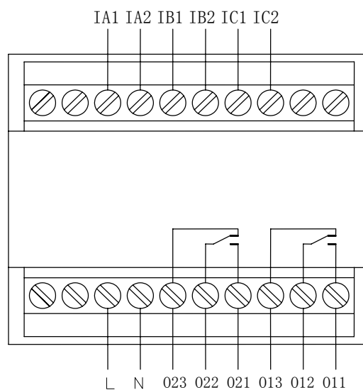
AMDS-□/B002 系列保护器主单元端子图
