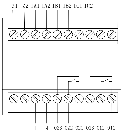
AMDS-□/B012 系列保护器主单元端子图
