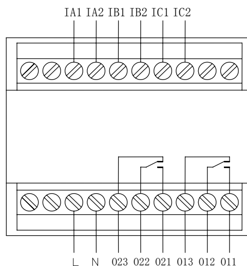
AMDS-□/D002、AMDS-□/D022 主单元端子图 AMDS-□/D032、AMDS-□/D042 主单元端子图
