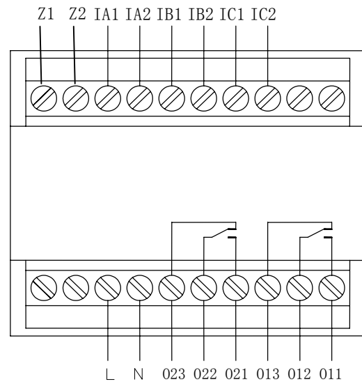
AMDS-□/D012、AMDS-□/D052 主单元端子图 AMDS-□/D062、AMDS-□/D072 主单元端子图
