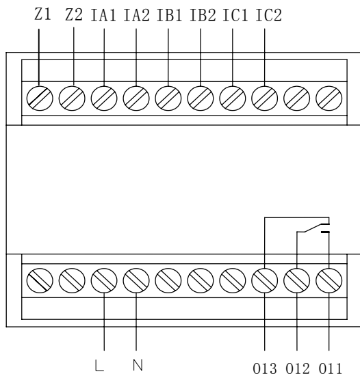
AMDS-□/D011、AMDS-□/D051 主单元端子图 AMDS-□/D061、AMDS-□/D071 主单元端子图
