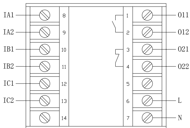
AMDT-□/C004、AMDT-□/C024 主单元端子图
