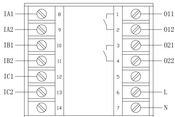
AMDT-□/C003、AMDT-□/C023 主单元端子图
