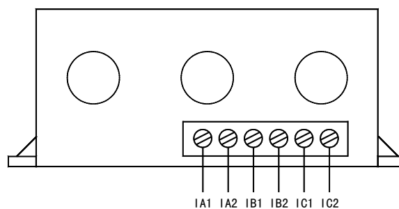
AMDT-□/C 系列电流检测单元接线端子图
