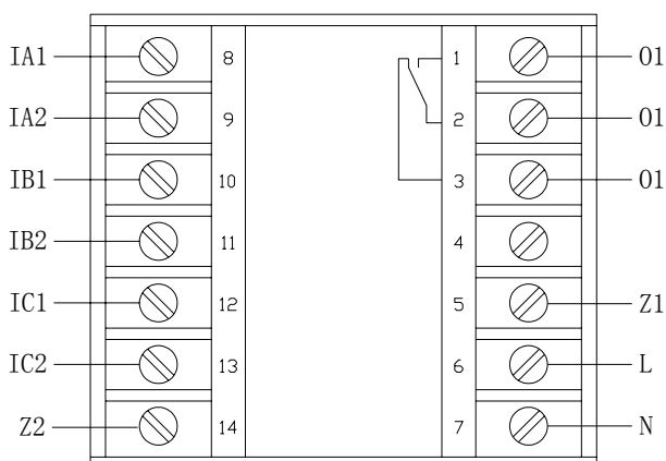
AMDT-□/C011、AMDT-□/C051 主单元端子图
