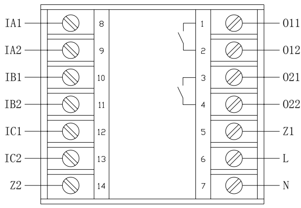
AMDT-□/C013、AMDT-□/C053 主单元端子图
