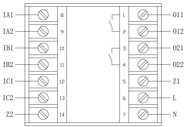
AMDT-X/E013、AMDT-X/E053 主单元端子图
