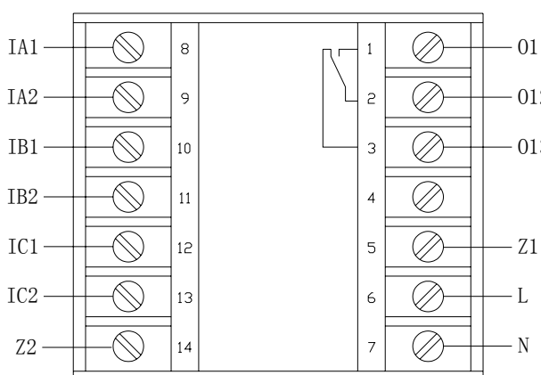
AMDT-X/E011、AMDT-X/E051 主单元端子图
