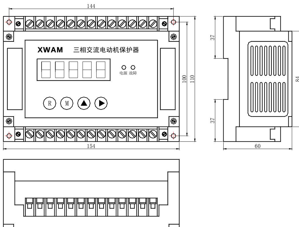
AMDG-□/CO 系列电动机保护器主单元外形及安装孔尺寸
