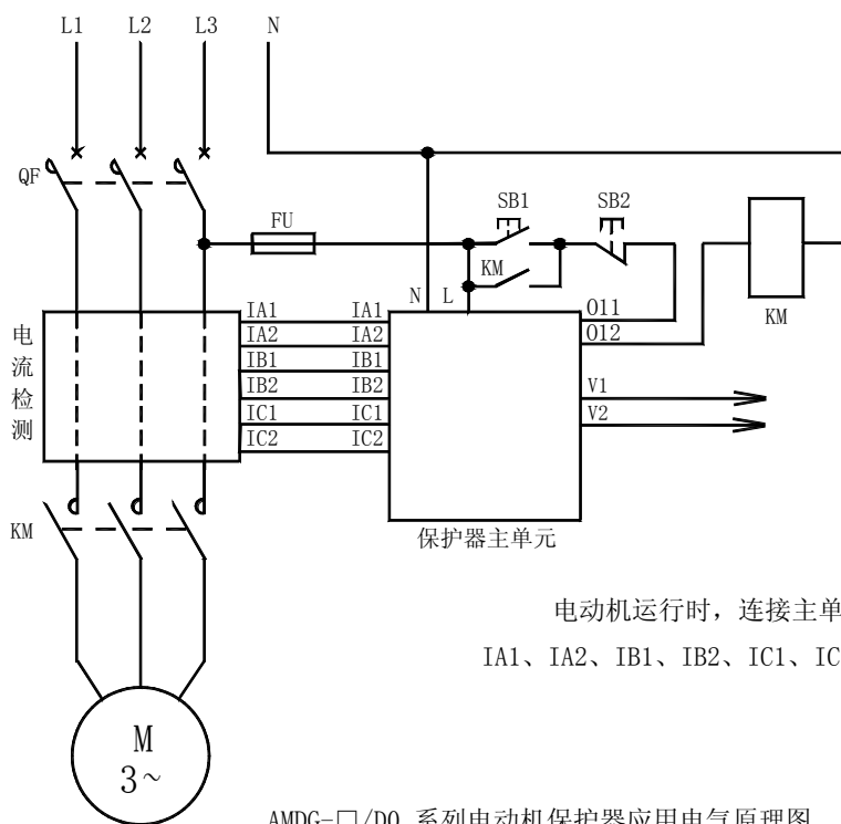
AMDG-□/DO 系列电动机保护器应用电气原理图
