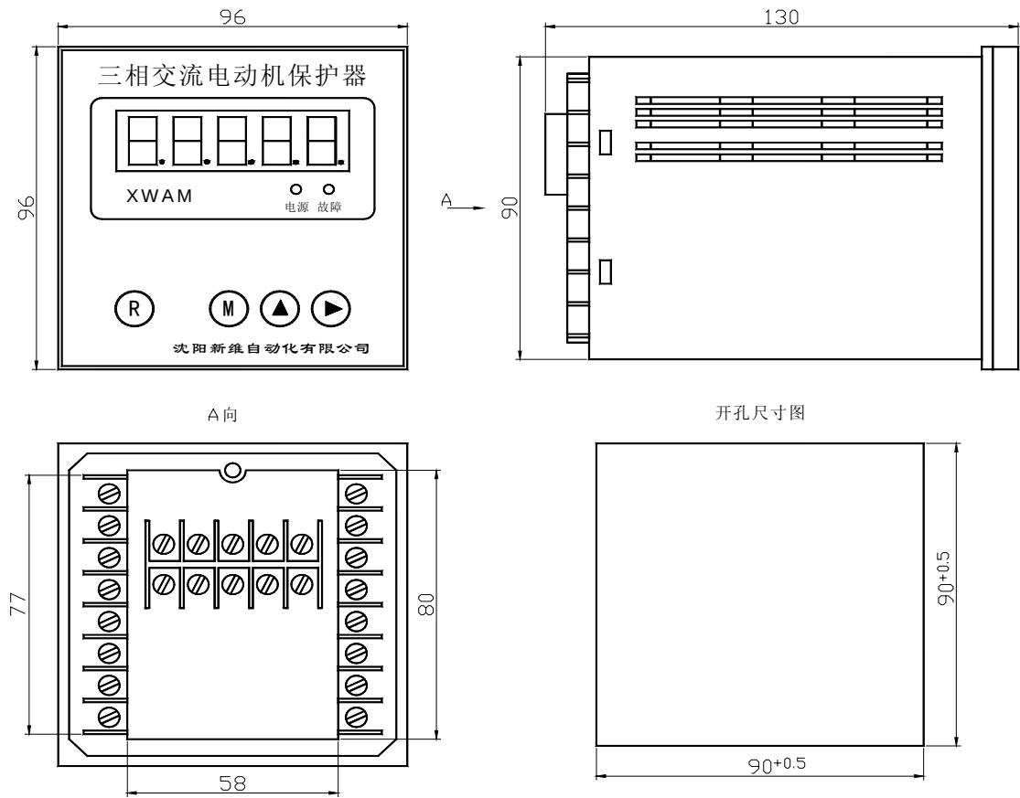
AMDP-□/D1 系列电动机保护器主单元外形及安装孔尺寸
