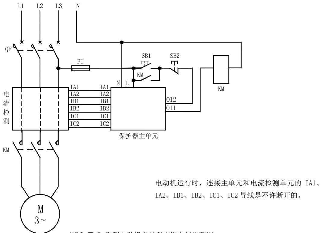
AMDS-□/B 系列电动机保护器应用电气原理图
