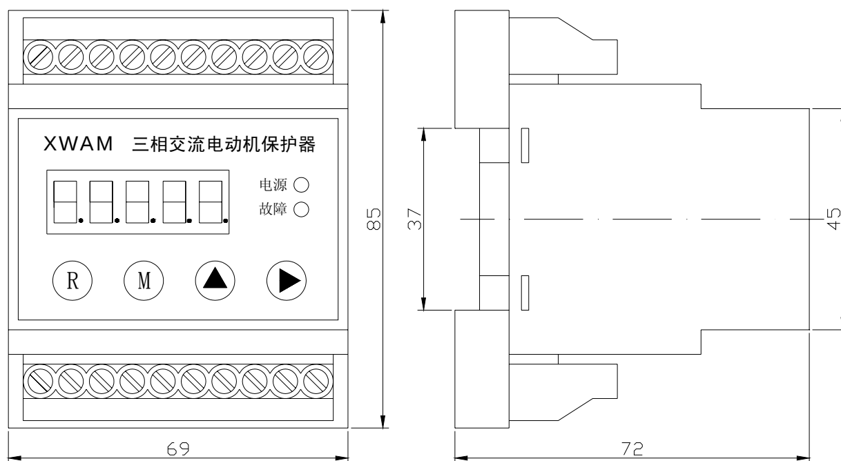
AMDS-□/D 系列电动机保护器主单元外形及安装孔尺寸
