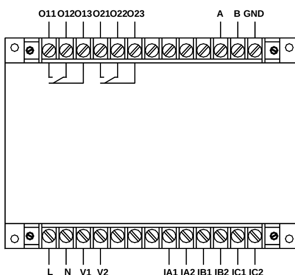
AMDG-□/D332 系列保护器主单元接线端子图
