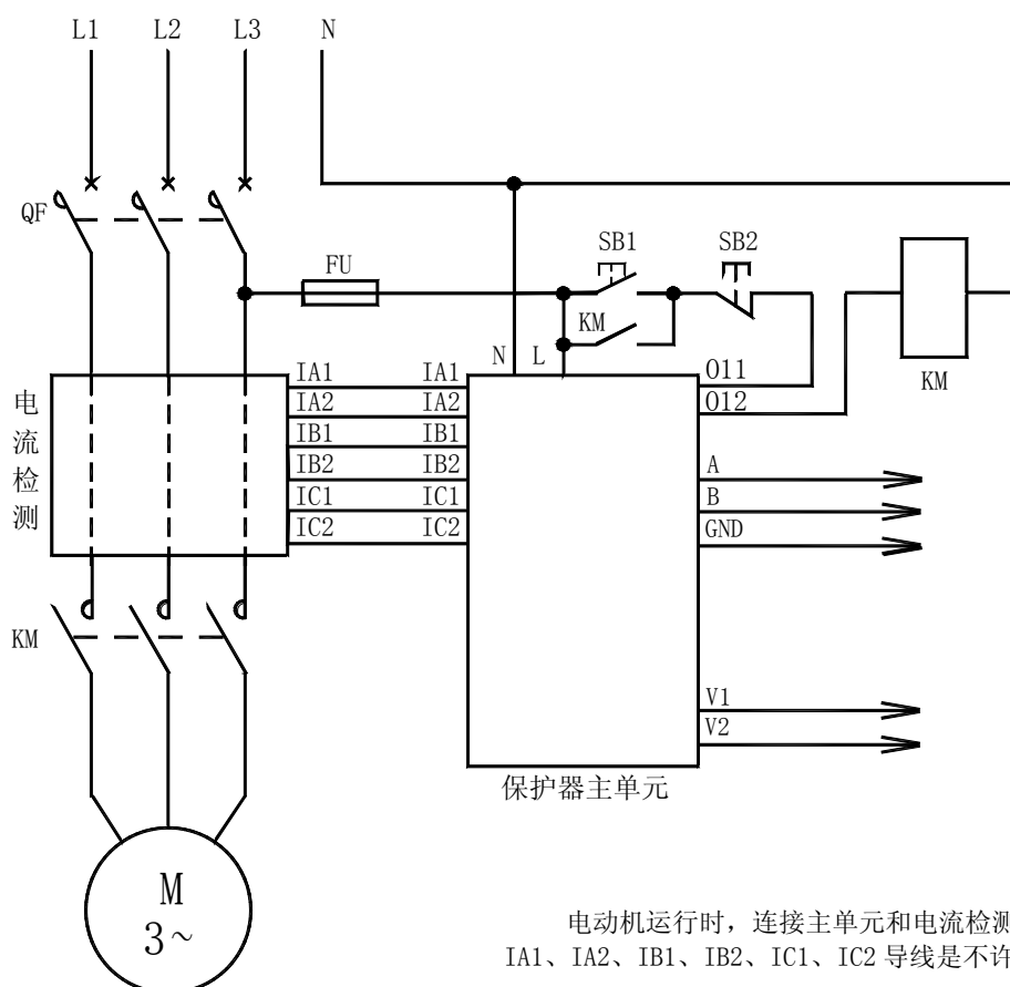
AMDG-□/D33□ 系列电动机保护器应用电气原理图
