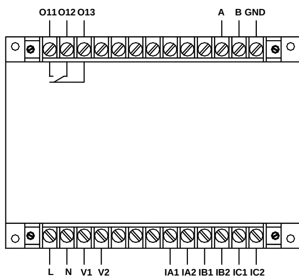
AMDG-□/D331 系列保护器主单元接线端子图
