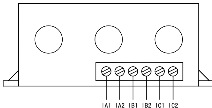
AMDG-□/D33□ 系列保护器电流检测单元接线端子图
