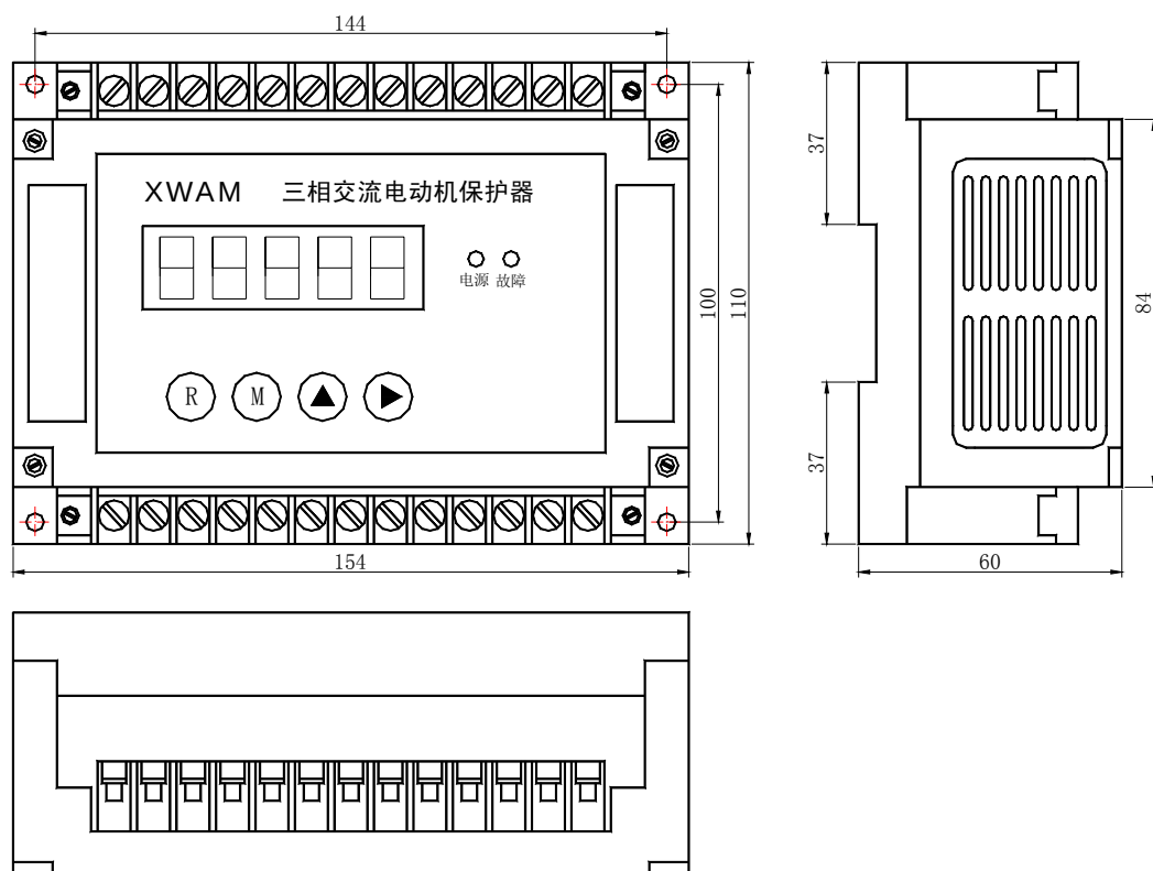
AMDG-□/ D801 系列电动机保护器主单元外形及安装孔尺寸
