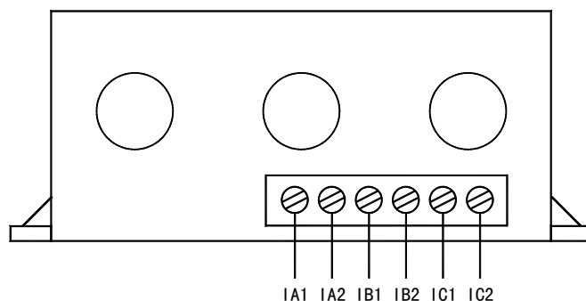
AMDG-□/D801 系列保护器电流检测单元接线端子图
