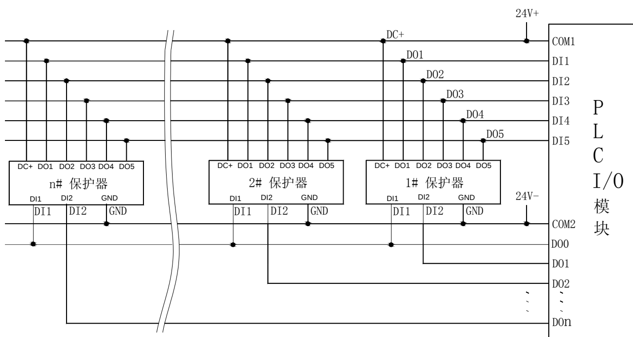
PLC 读取多台 AMDG-□/D801 系列电动机保护器电气原理图
