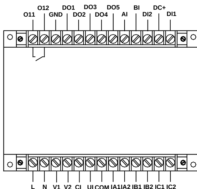
AMDG-□/D801 系列保护器主单元接线端子图
