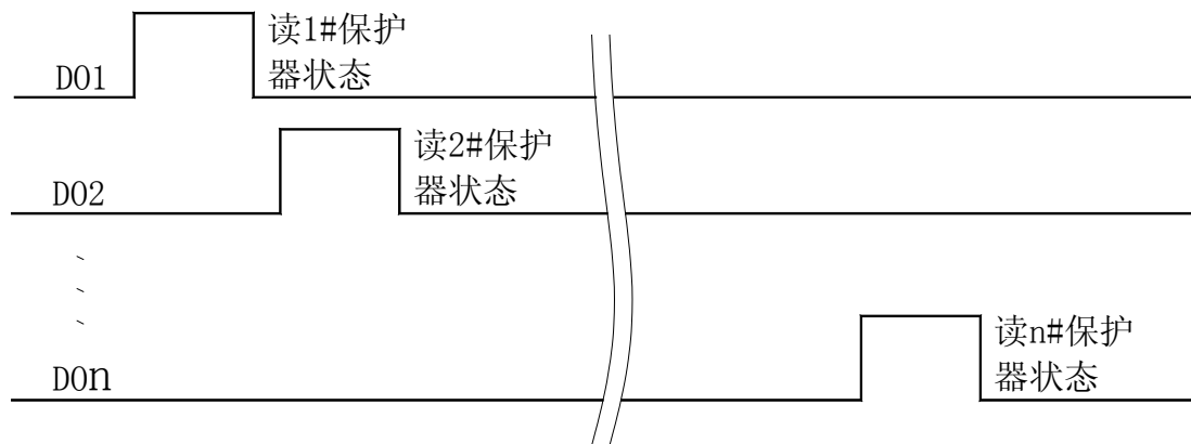
PLC 读取多台 AMDG-□/D801 系列电动机保护器时序图
