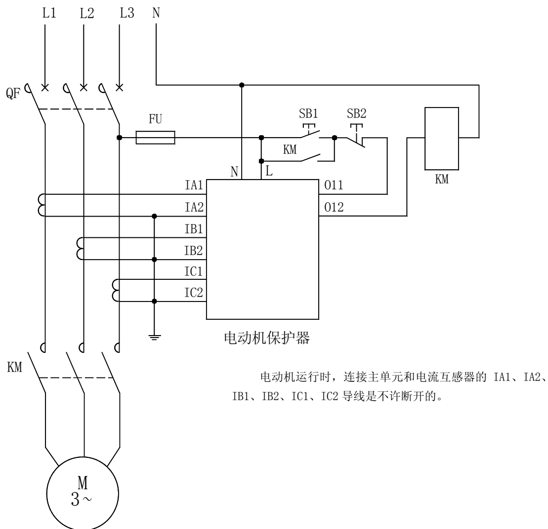
AMDG-X/E00□ 系列电动机保护器应用电气原理图
