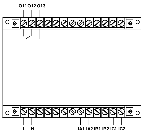
AMDG-X/E001 系列保护器主单元接线端子图
