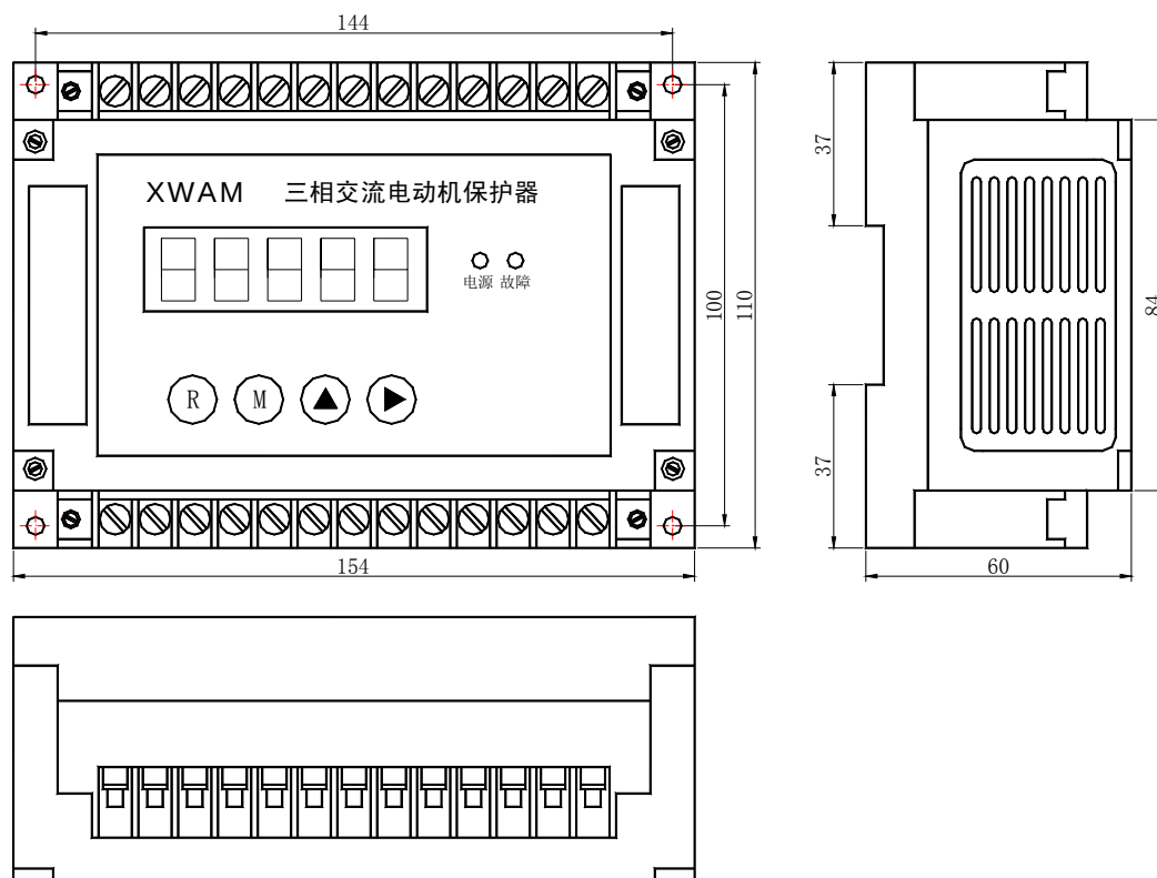
AMDG-X/E00□ 系列电动机保护器主单元外形及安装孔尺寸
