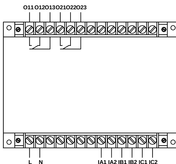
AMDG-X/E002 系列保护器主单元接线端子图
