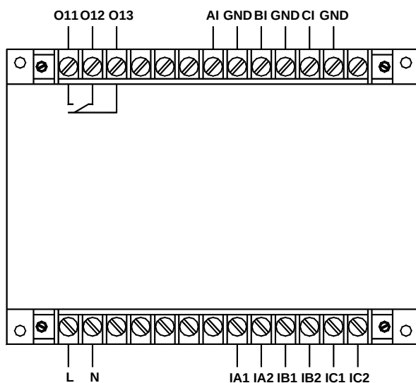
AMDG-X/E121 系列保护器主单元接线端子图
