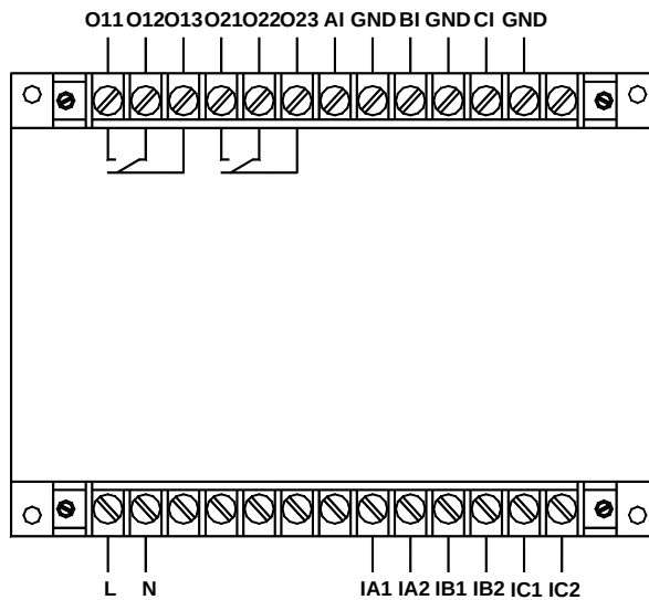
AMDG-X/E122 系列保护器主单元接线端子图
