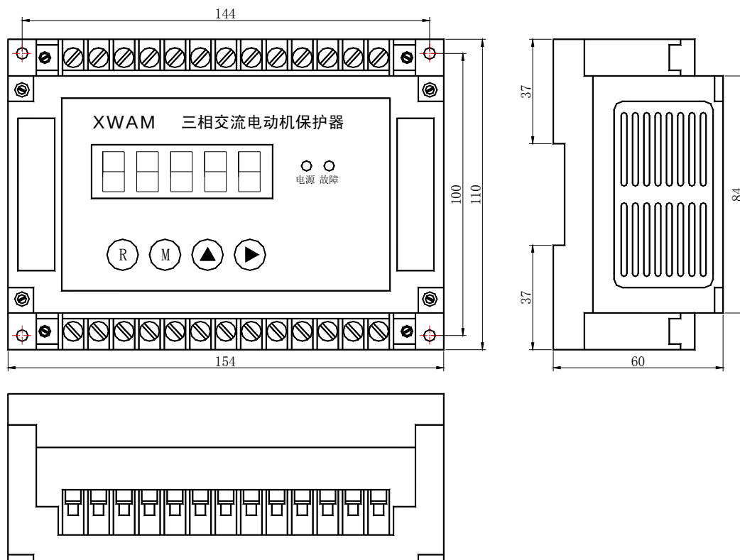
AMDG-X/E12□ 系列电动机保护器主单元外形及安装孔尺寸
