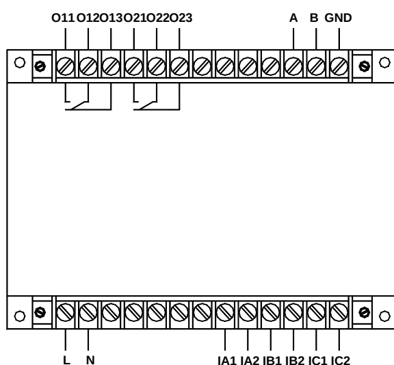
AMDG-X/E322 系列保护器主单元接线端子图
