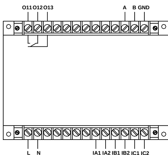
AMDG-X/E321 系列保护器主单元接线端子图
