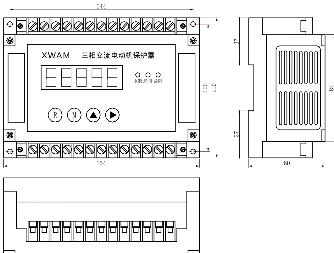
AMDG-X/E32□ 系列电动机保护器主单元外形及安装孔尺寸
