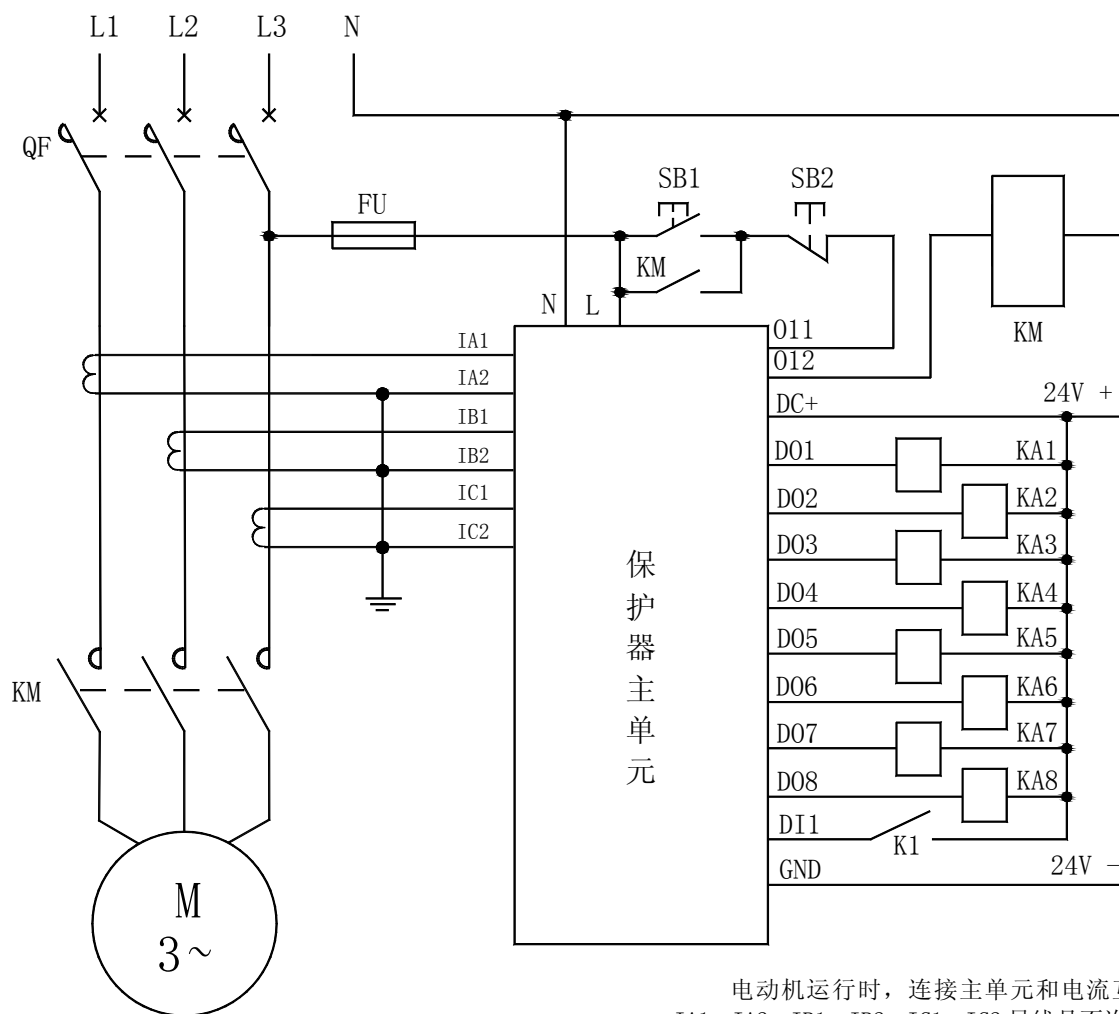
AMDG-X/E501 系列电动机保护器 D0 连接继电器电气原理图
