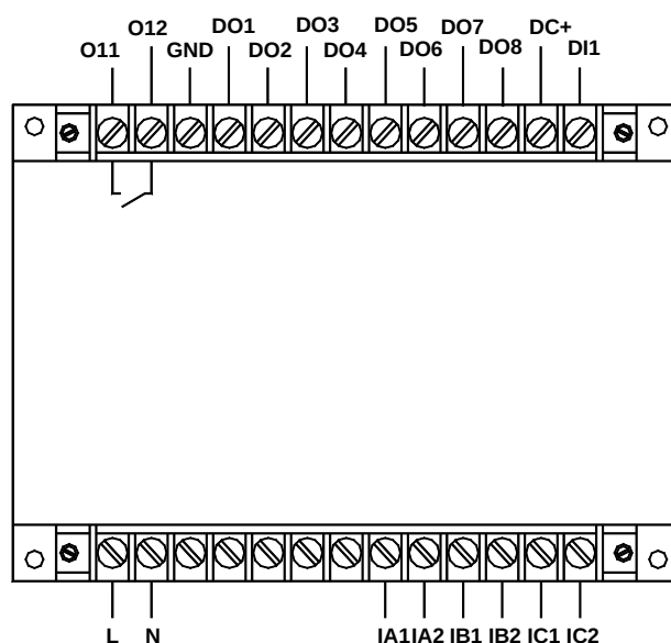
AMDG-X/E501 系列保护器主单元接线端子图
