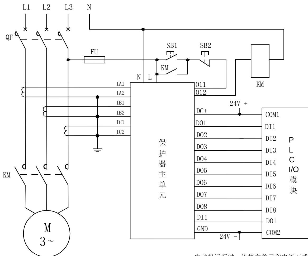
AMDG-X/E501 系列电动机保护器 D0 连接 PLC 电气原理图
