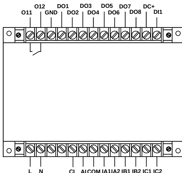
AMDG-X/E721 系列保护器主单元接线端子图
