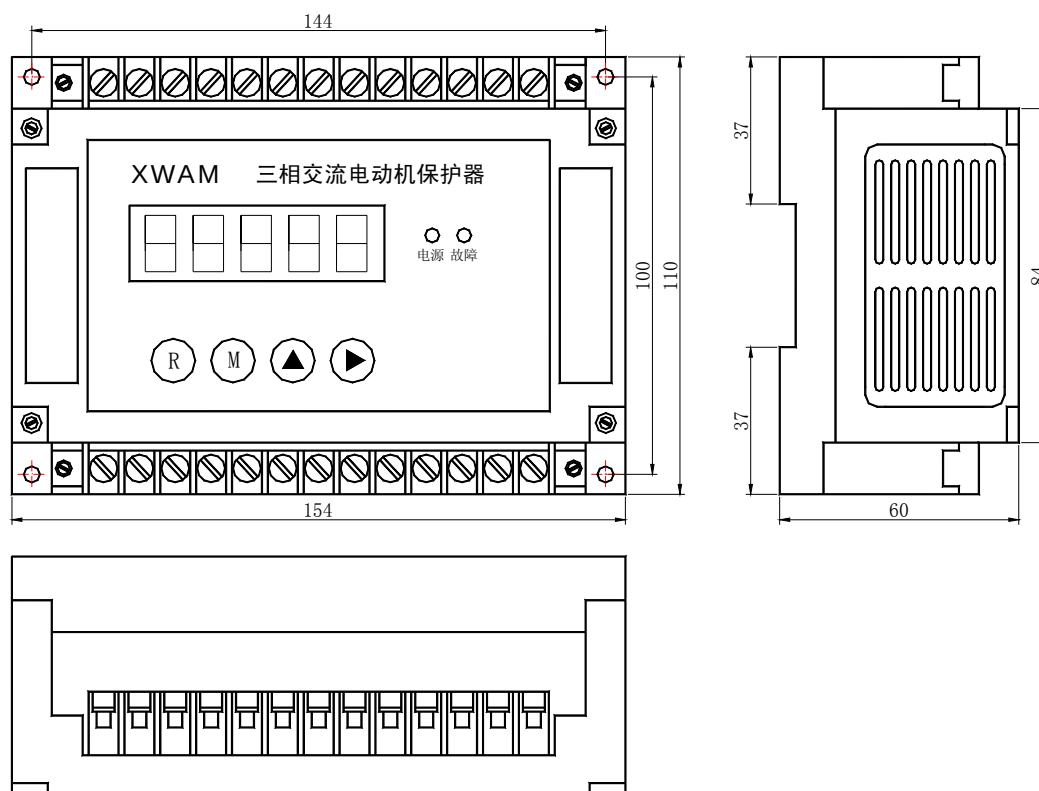
AMDG-X/E721 系列电动机保护器主单元外形及安装孔尺寸
