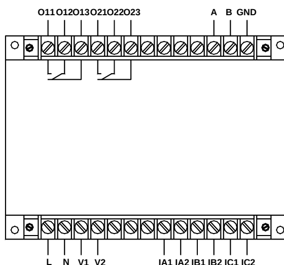
AMDG-X/F322 系列保护器主单元接线端子图
