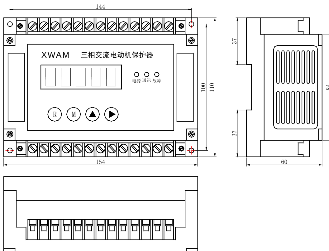
AMDG-X/F32□ 系列电动机保护器主单元外形及安装孔尺寸
