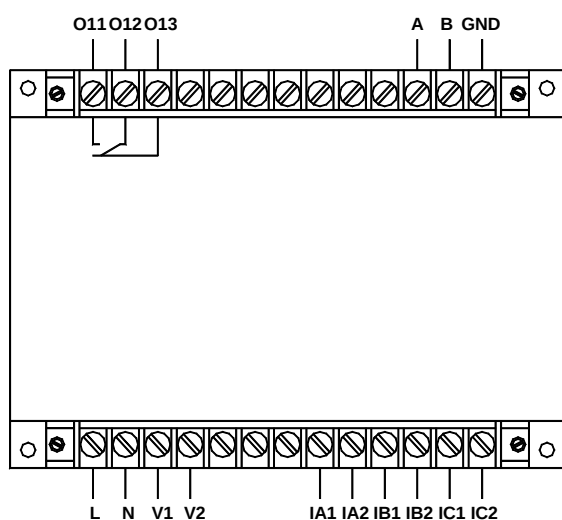
AMDG-X/F321 系列保护器主单元接线端子图
