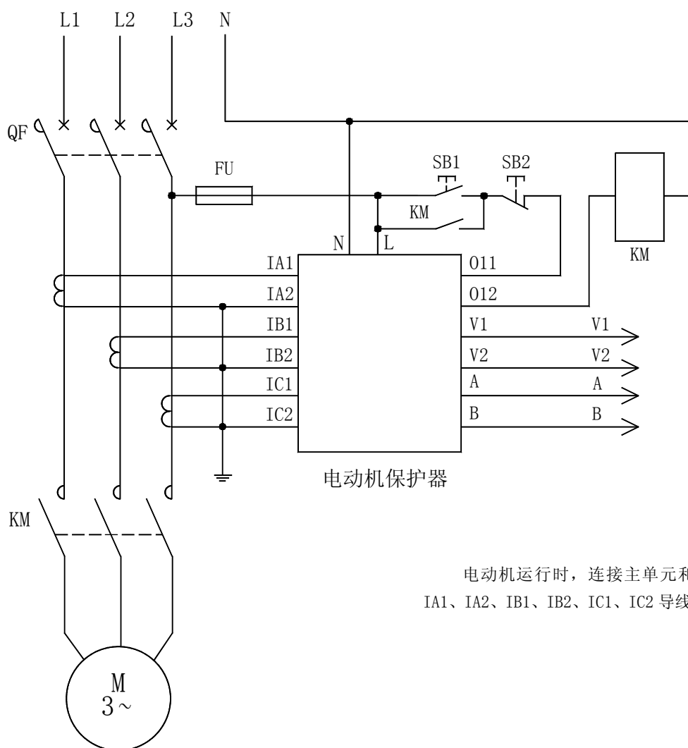
AMDG-X/F32□ 系列电动机保护器应用电气原理图
