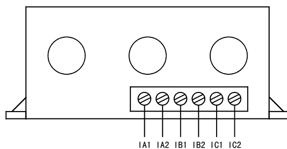
AMDGH-□/C41□ 系列保护器电流检测单元接线端子图
