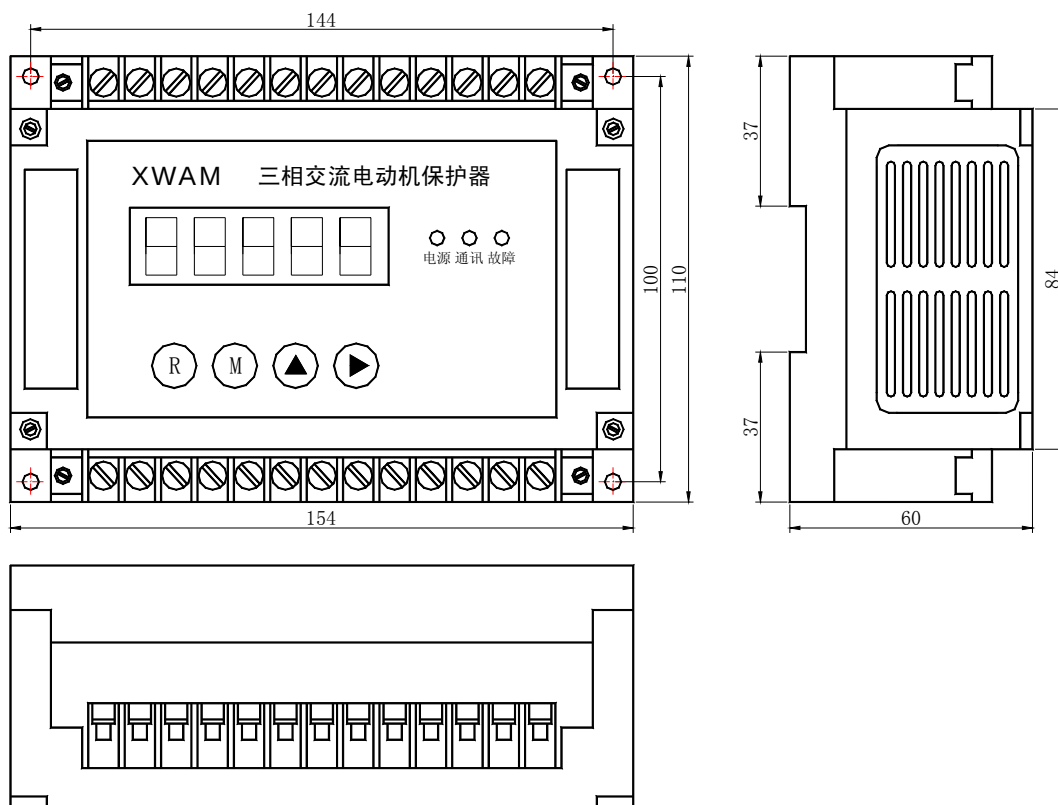
AMDGH-□/C41□ 系列电动机保护器主单元外形及安装孔尺寸
