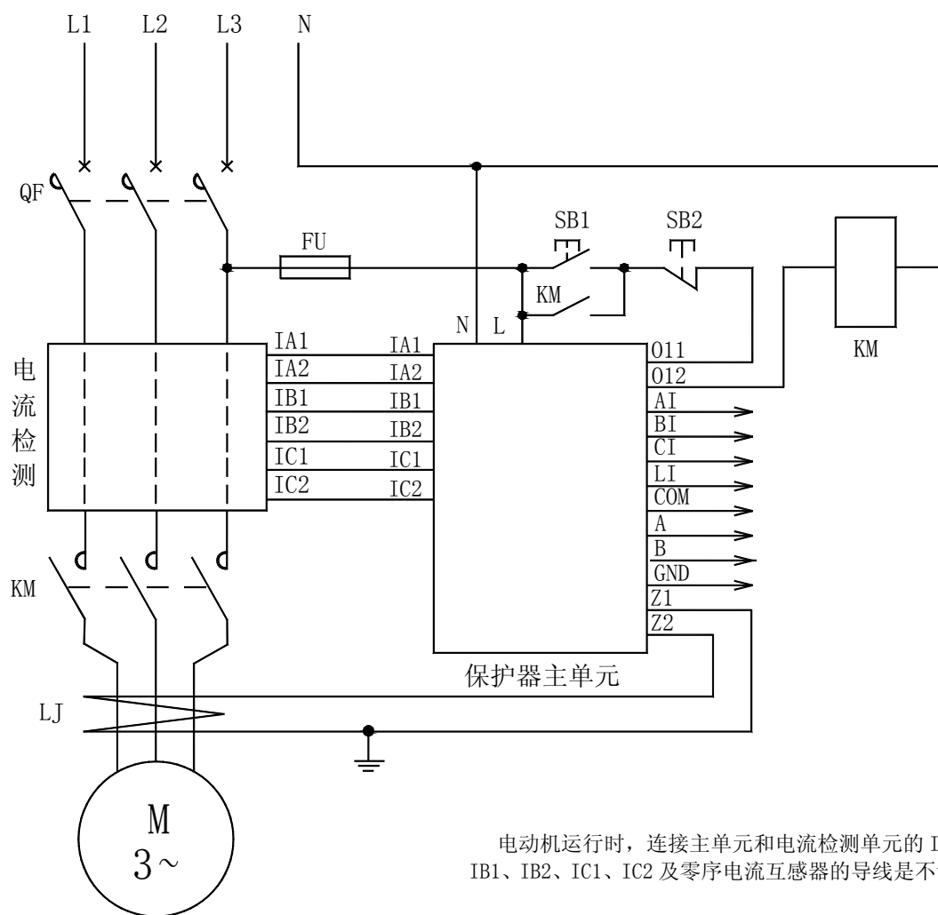
AMDGH-□/C41□ 系列电动机保护器应用电气原理图
