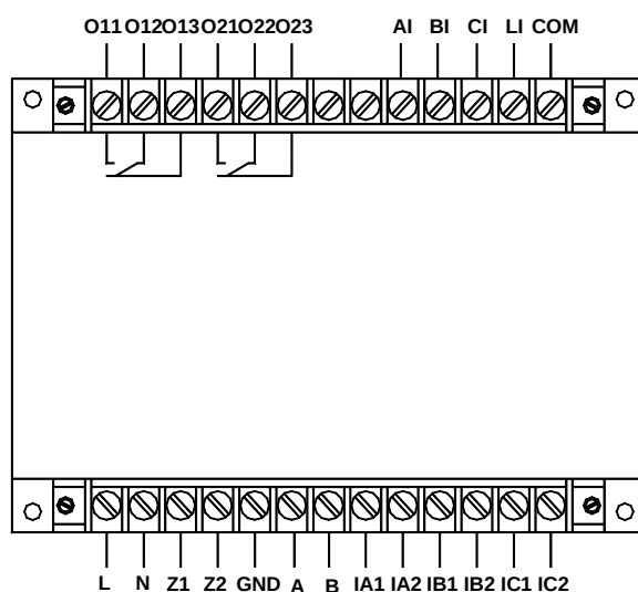
AMDGH-□/□C412 系列保护器主单元接线端子图
