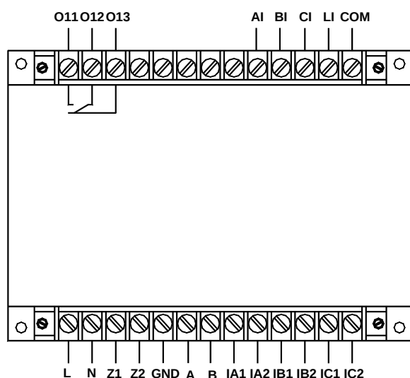
AMDGH-□/□C411 系列保护器主单元接线端子图
