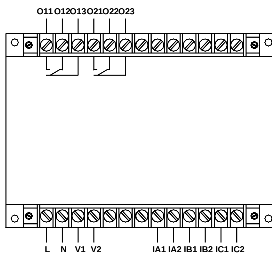
AMDGH-□/D002 系列保护器主单元接线端子图
