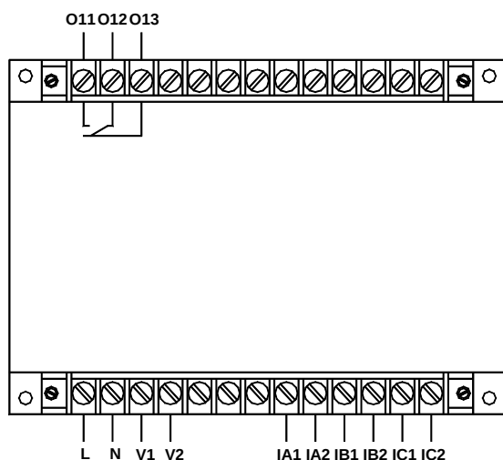
AMDGH-□/D001 系列保护器主单元接线端子图
