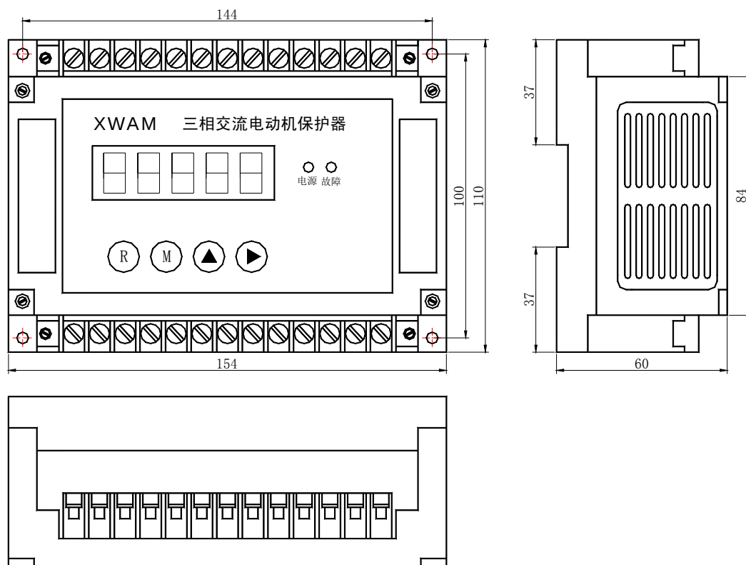
AMDGH-□/DO0□ 系列电动机保护器主单元外形及安装孔尺寸
