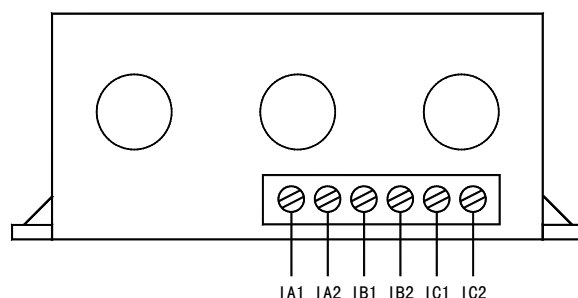
AMDGH-□/DO0□ 系列保护器电流检测单元接线端子图
