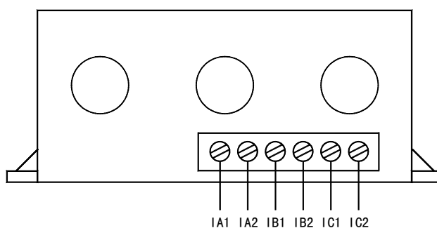
AMDGH-□/D01□ 系列保护器电流检测单元接线端子图
