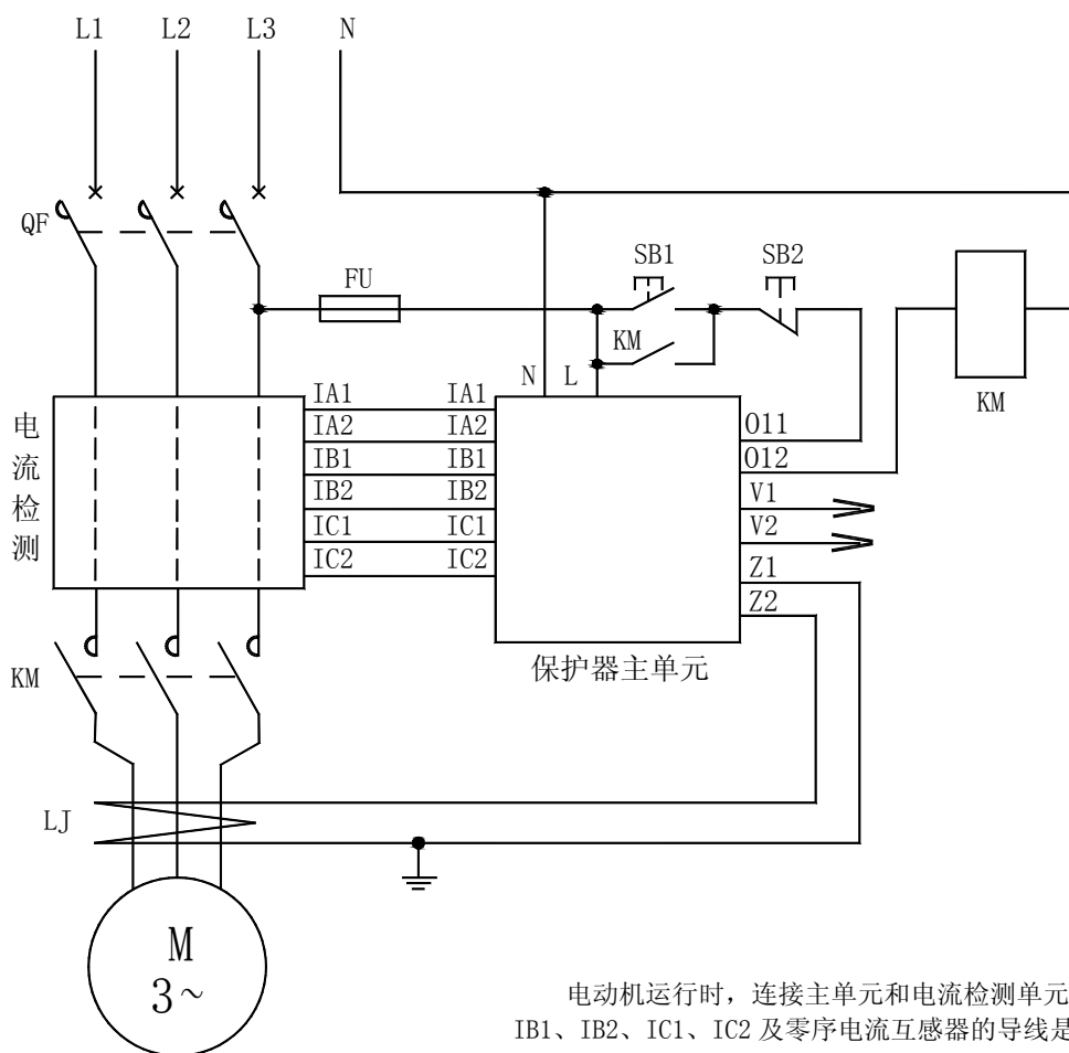
AMDGH-□/D01□ 系列电动机保护器应用电气原理图
