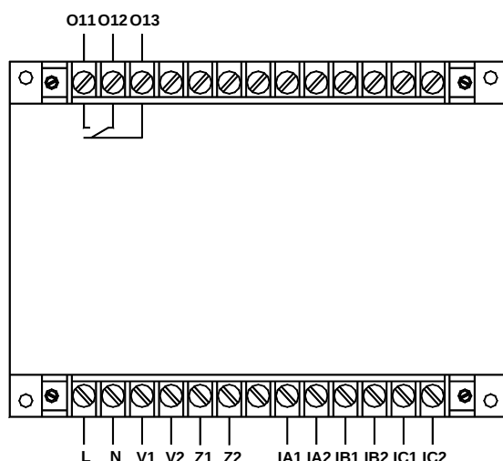
AMDGH-□/D011 系列保护器主单元接线端子图
