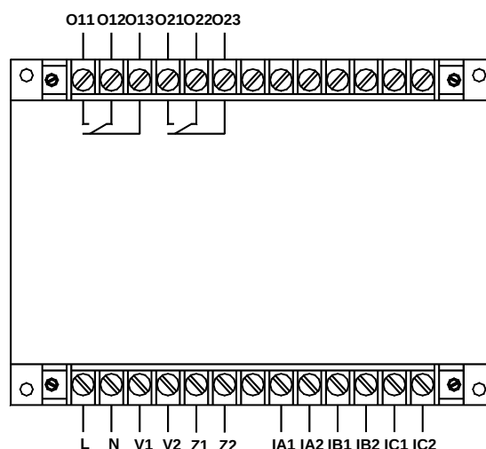
AMDGH-□/D012 系列保护器主单元接线端子图
