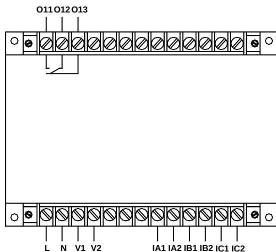
AMDGH-□/D021 系列保护器主单元接线端子图
