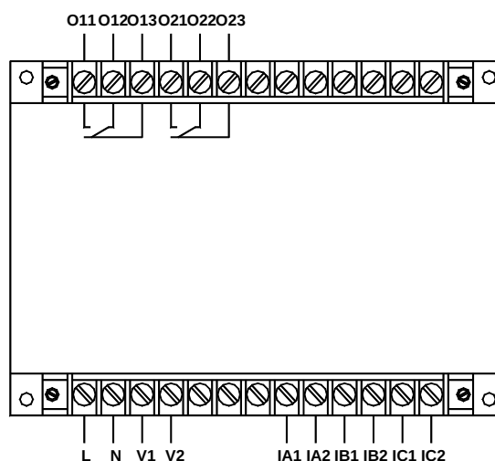
AMDGH-□/D022 系列保护器主单元接线端子图
