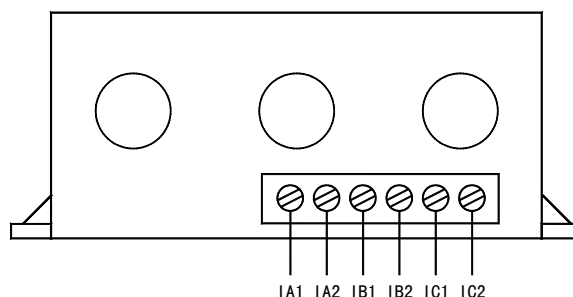
AMDGH-□/D02□ 系列保护器电流检测单元接线端子图
