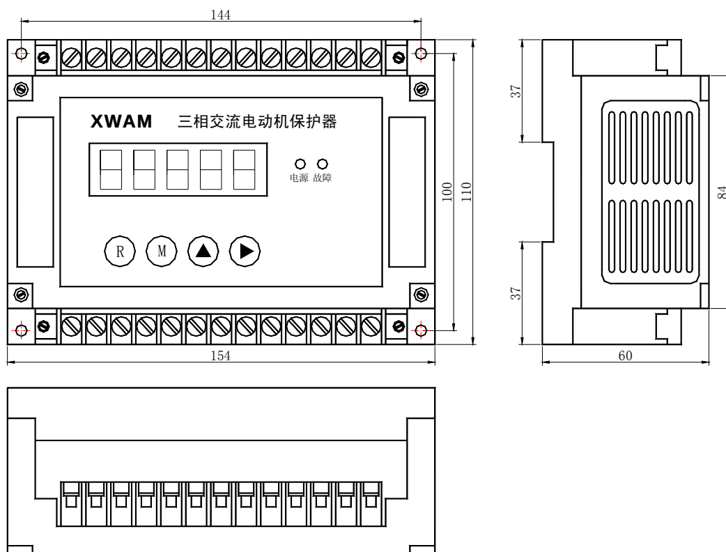
AMDGH-□/DO2□ 系列电动机保护器主单元外形及安装孔尺寸
