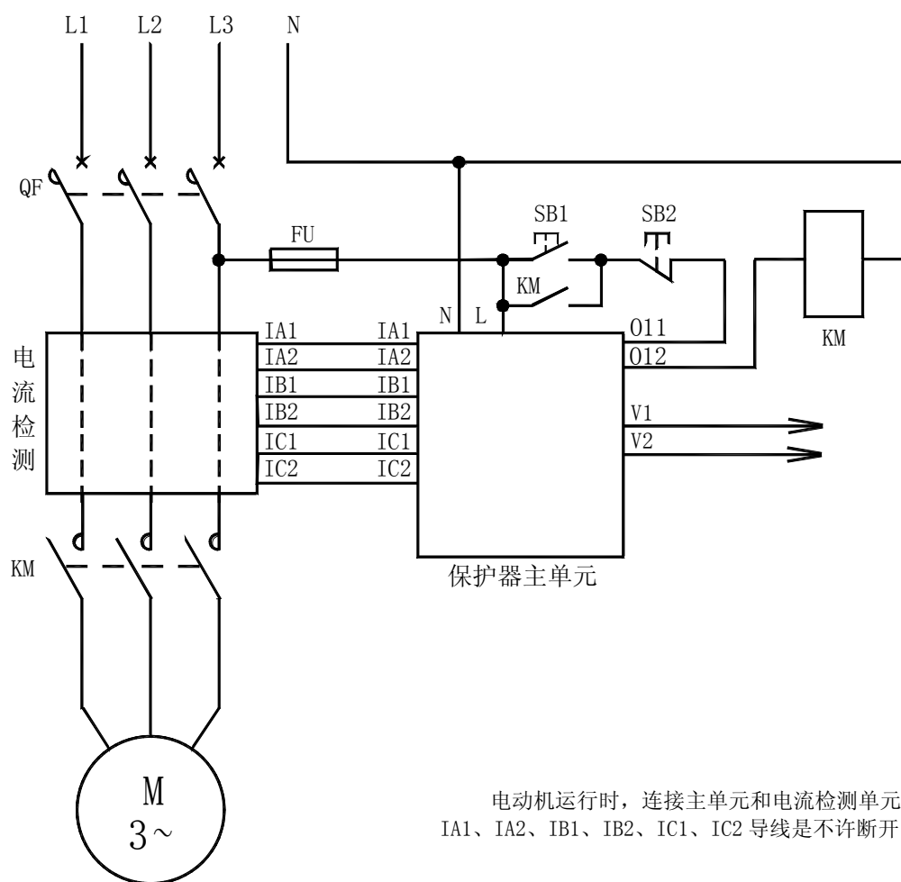
AMDGH-□/D02□ 系列电动机保护器应用电气原理图
