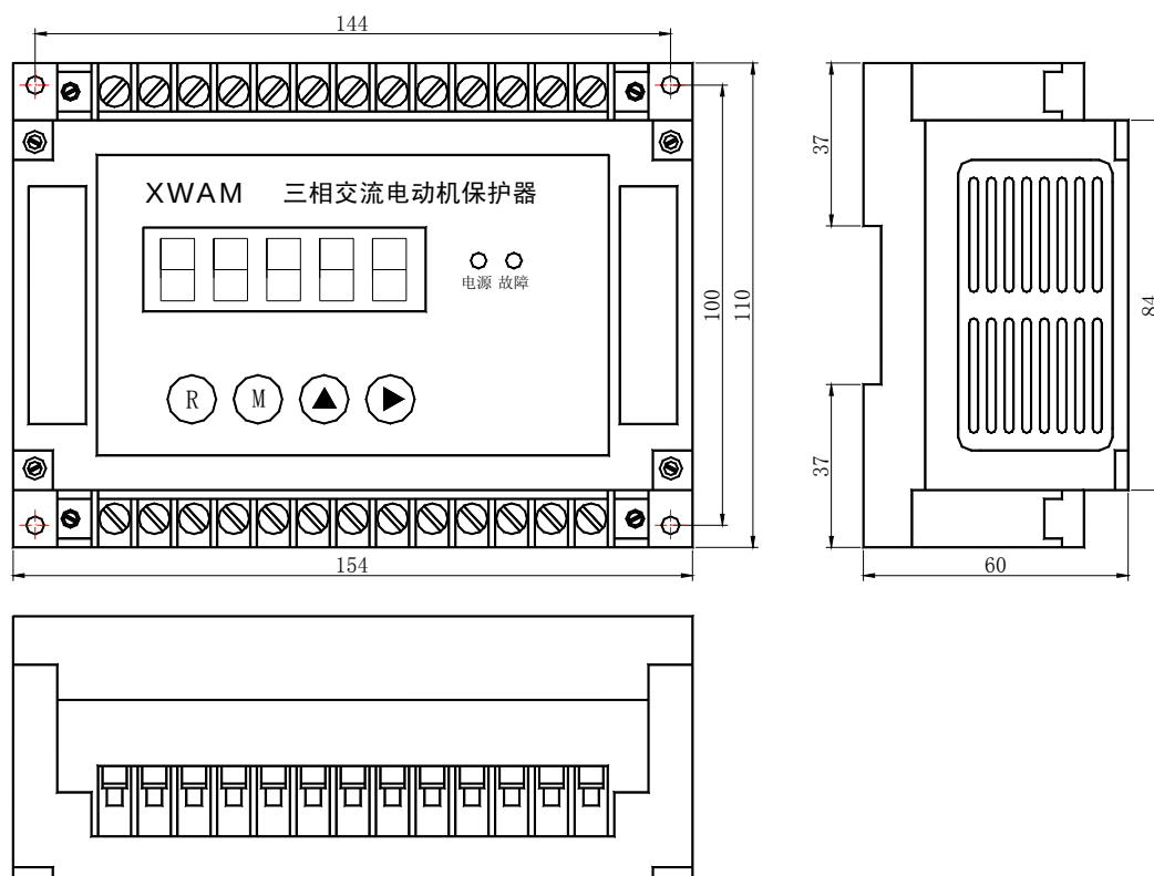
AMDGH-□/D03□ 系列电动机保护器主单元外形及安装孔尺寸
