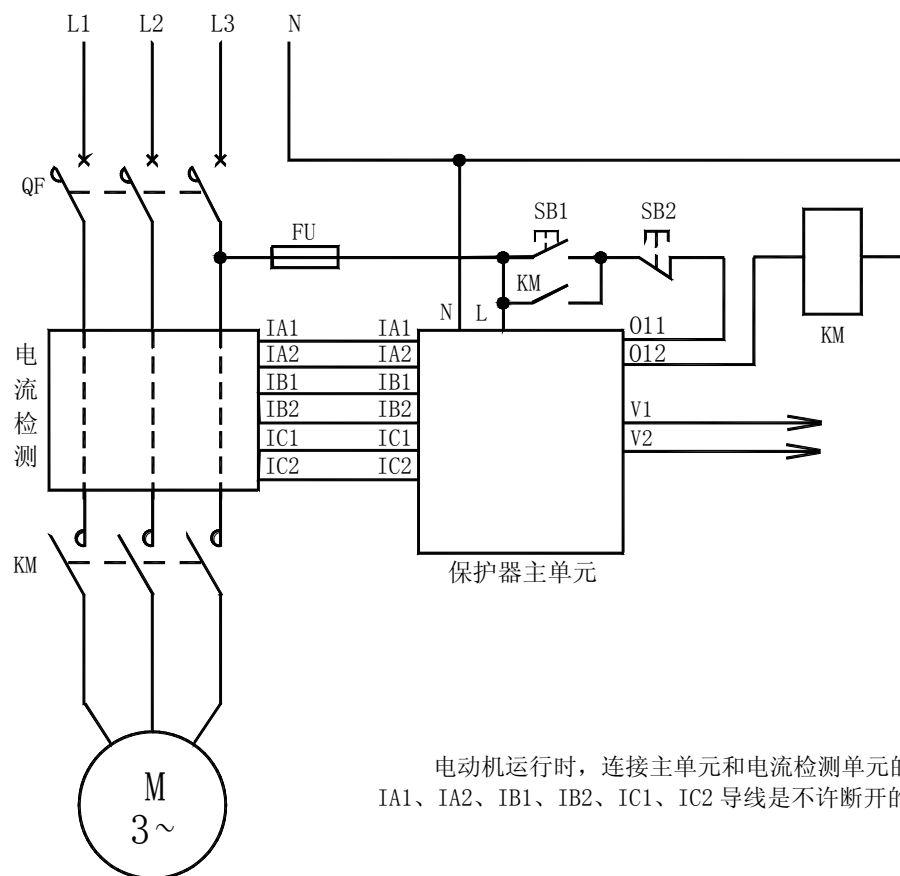
AMDGH-□/D03□ 系列电动机保护器应用电气原理图
