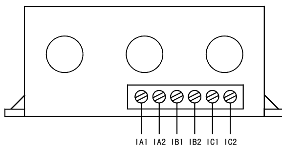
AMDGH-□/D03□ 系列保护器电流检测单元接线端子图
