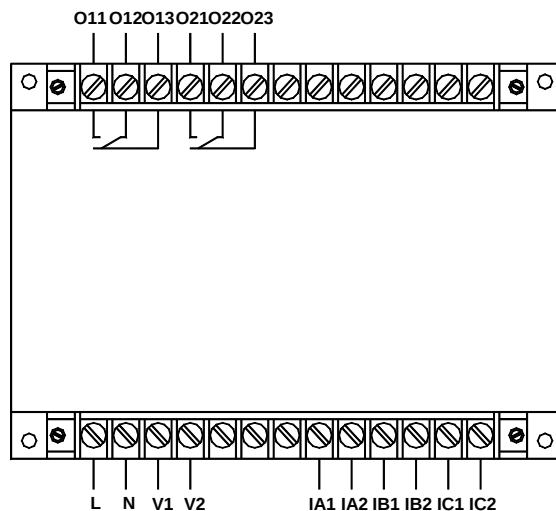
AMDGH-□/D032 系列保护器主单元接线端子图
