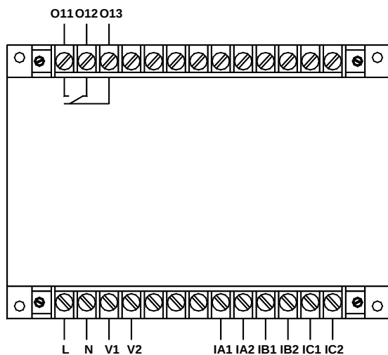
AMDGH-□/D031 系列保护器主单元接线端子图
