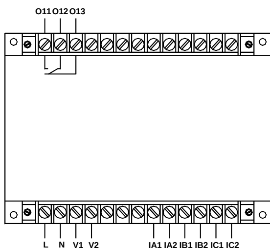
AMDGH-□/D041 系列保护器主单元接线端子图
