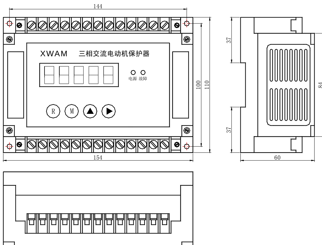
AMDGH-□/DO4□ 系列电动机保护器主单元外形及安装孔尺寸
