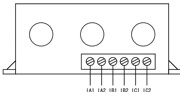
AMDGH-□/D04□ 系列保护器电流检测单元接线端子图
