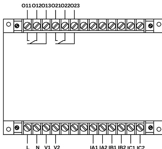
AMDGH-□/D042 系列保护器主单元接线端子图
