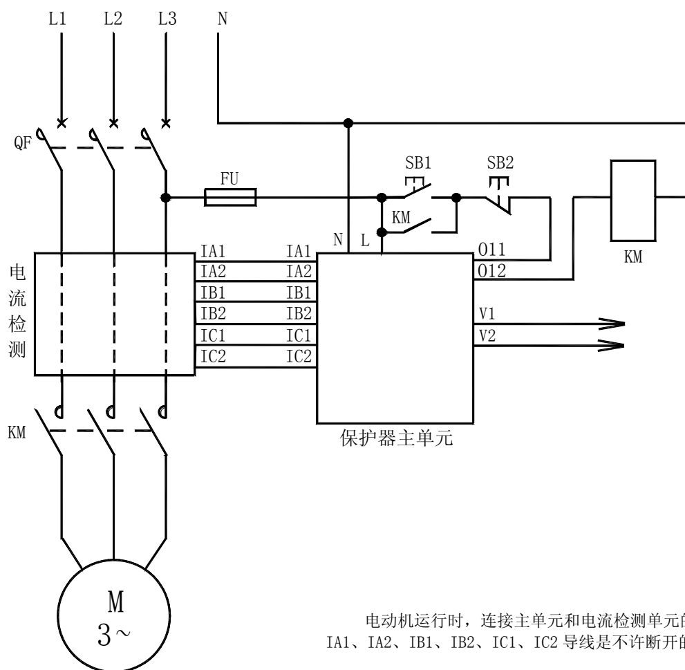
AMDGH-□/D04□ 系列电动机保护器应用电气原理图
