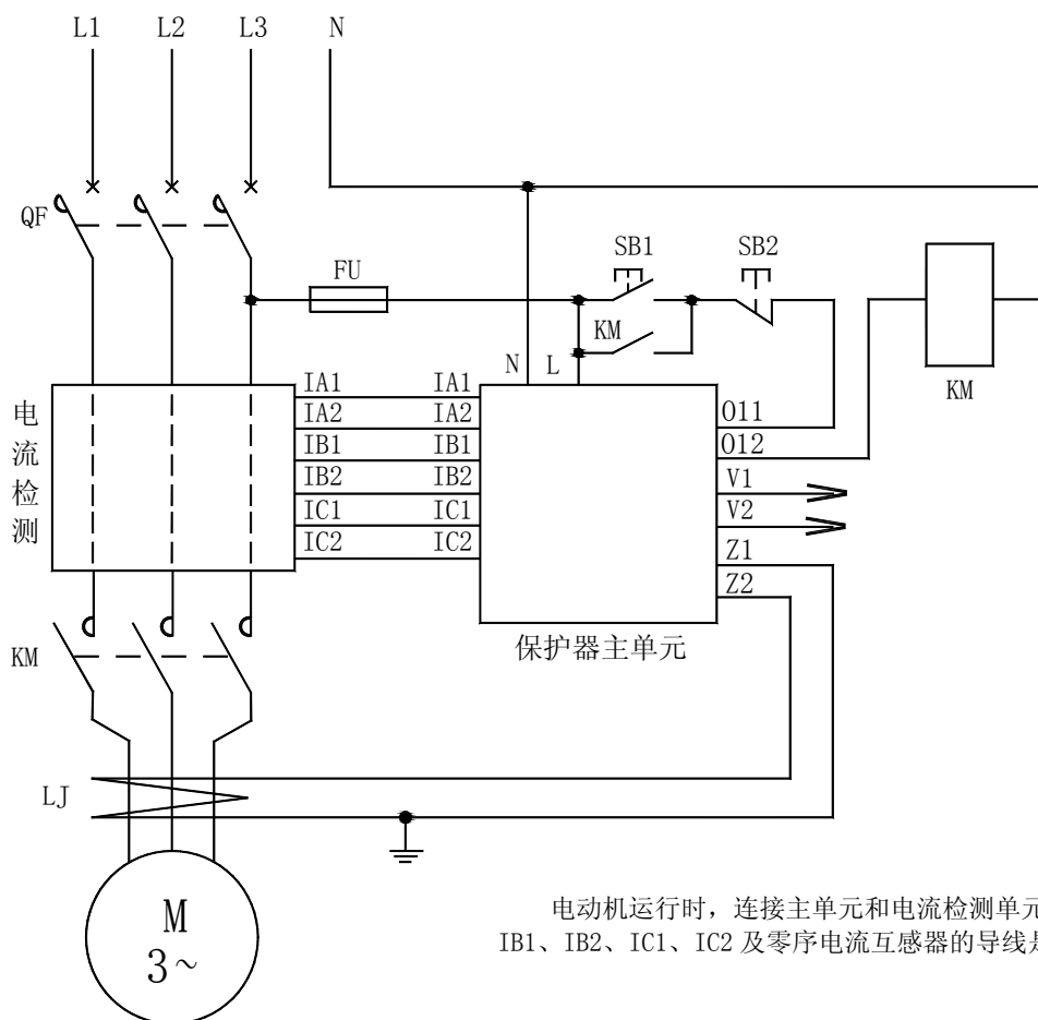
AMDGH-□/D05□ 系列电动机保护器应用电气原理图
