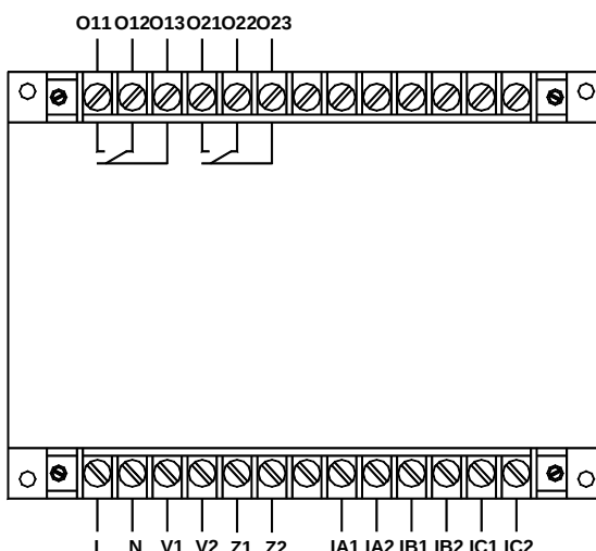
AMDGH-□/D052 系列保护器主单元接线端子图
