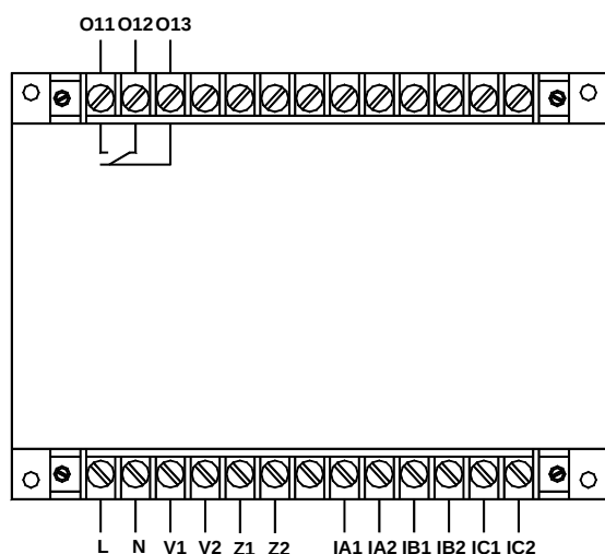
AMDGH-□/D051 系列保护器主单元接线端子图
