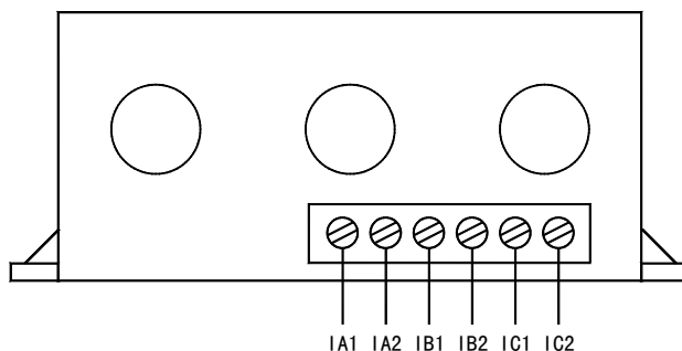
AMDGH-□/D05□ 系列保护器电流检测单元接线端子图
