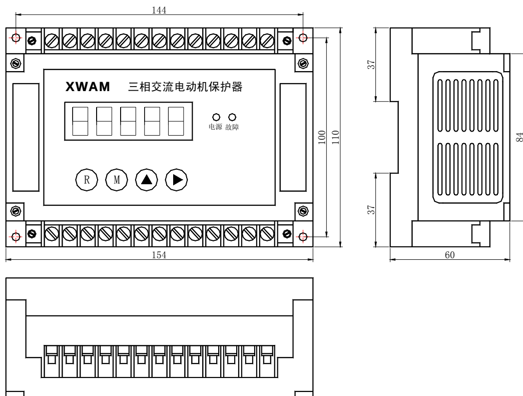
AMDGH-□/DO5□ 系列电动机保护器主单元外形及安装孔尺寸
