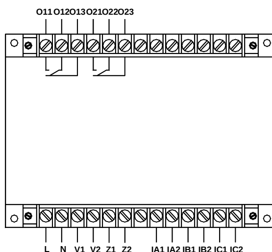
AMDGH-□/D062 系列保护器主单元接线端子图
