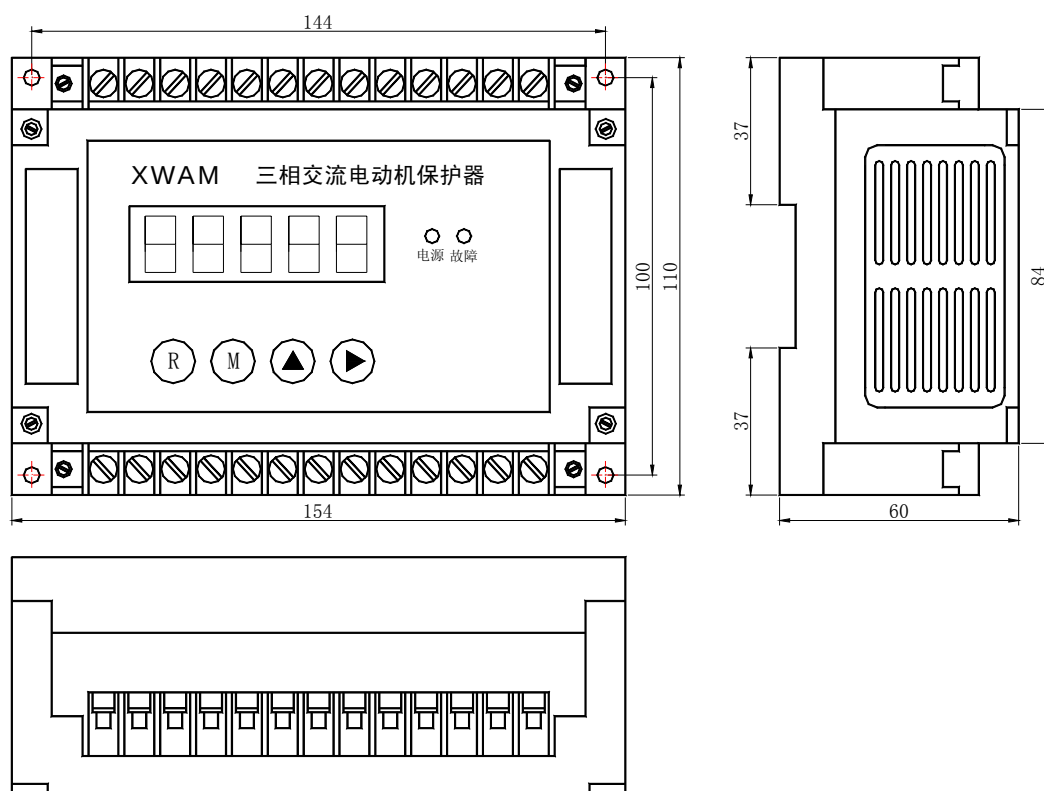
AMDGH-□/DO6□ 系列电动机保护器主单元外形及安装孔尺寸
