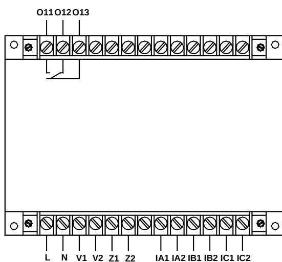
AMDGH-□/D061 系列保护器主单元接线端子图
