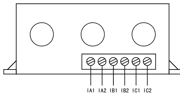
AMDGH-□/D06□ 系列保护器电流检测单元接线端子图
