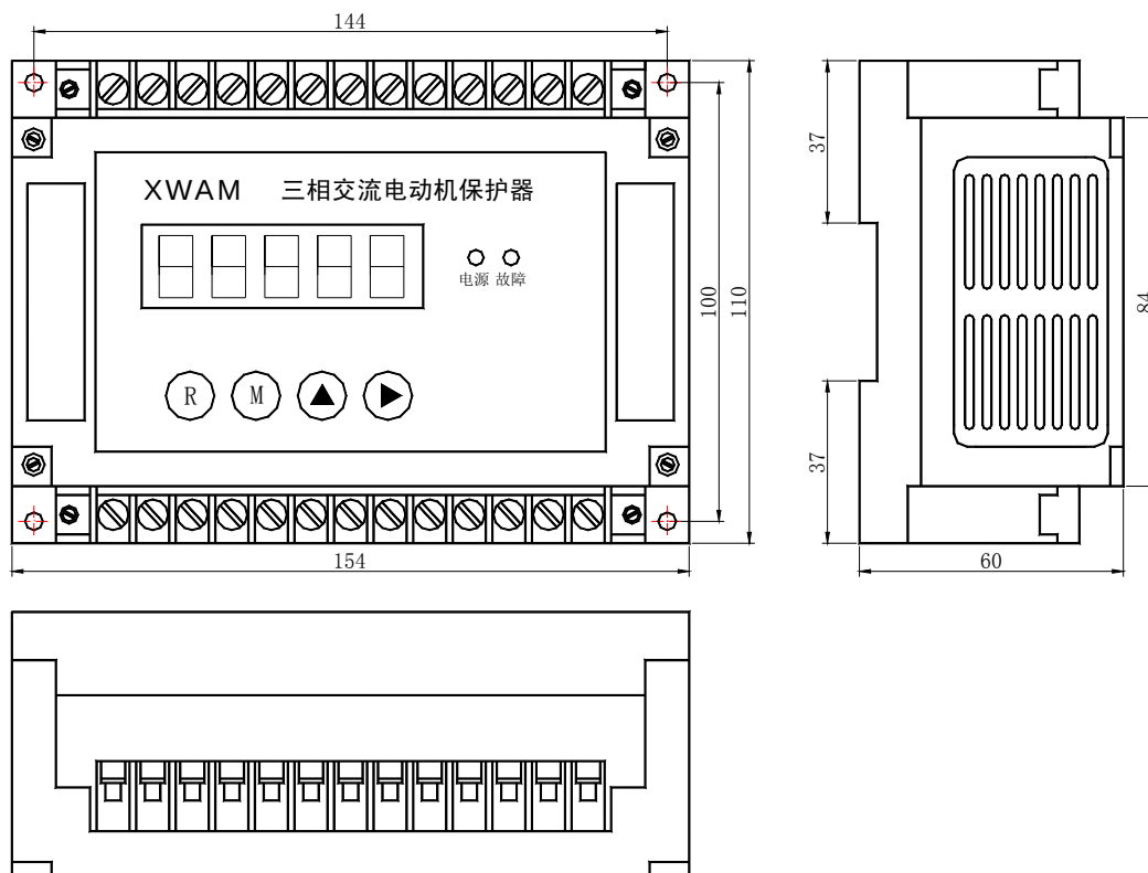
AMDGH-□/DO7□ 系列电动机保护器主单元外形及安装孔尺寸
