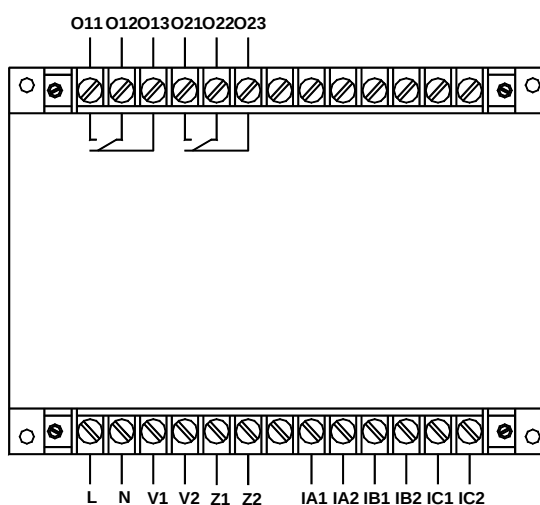
AMDGH-□/D072 系列保护器主单元接线端子图
