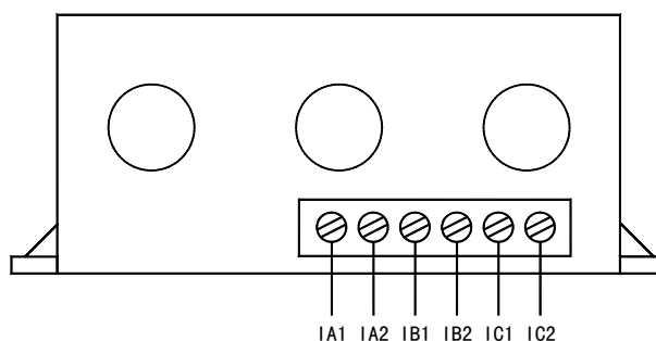
AMDGH-□/D07□ 系列保护器电流检测单元接线端子图
