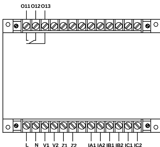
AMDGH-□/D071 系列保护器主单元接线端子图
