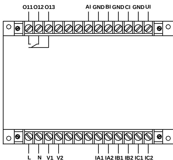
AMDGH-□/D101 系列保护器主单元接线端子图
