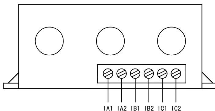
AMDGH-□/D10□ 系列保护器电流检测单元接线端子图
