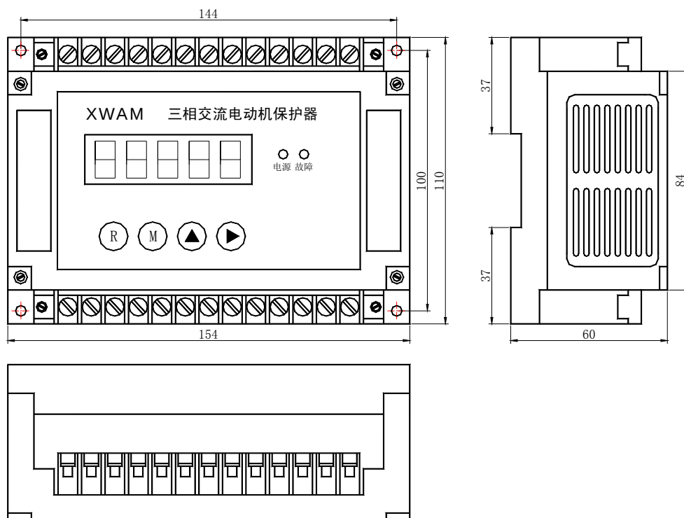
AMDGH-□/D10□ 系列电动机保护器主单元外形及安装孔尺寸
