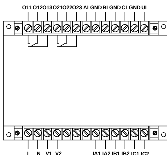
AMDGH-□/D102 系列保护器主单元接线端子图
