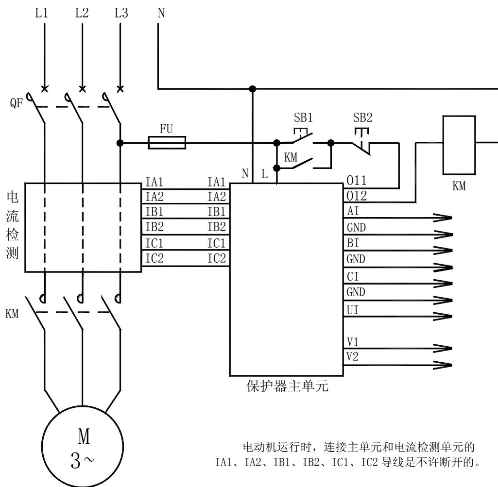
AMDGH-□/D10□ 系列电动机保护器应用电气原理图
