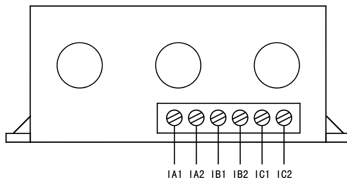
AMDGH-□/D11□ 系列保护器电流检测单元接线端子图
