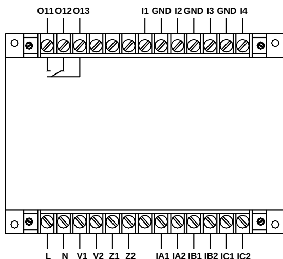
AMDGH-□/D111 系列保护器主单元接线端子图
