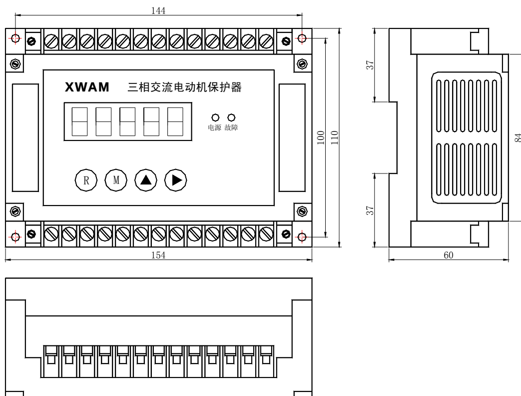
AMDGH-□/□/D11□ 系列电动机保护器主单元外形及安装孔尺寸
