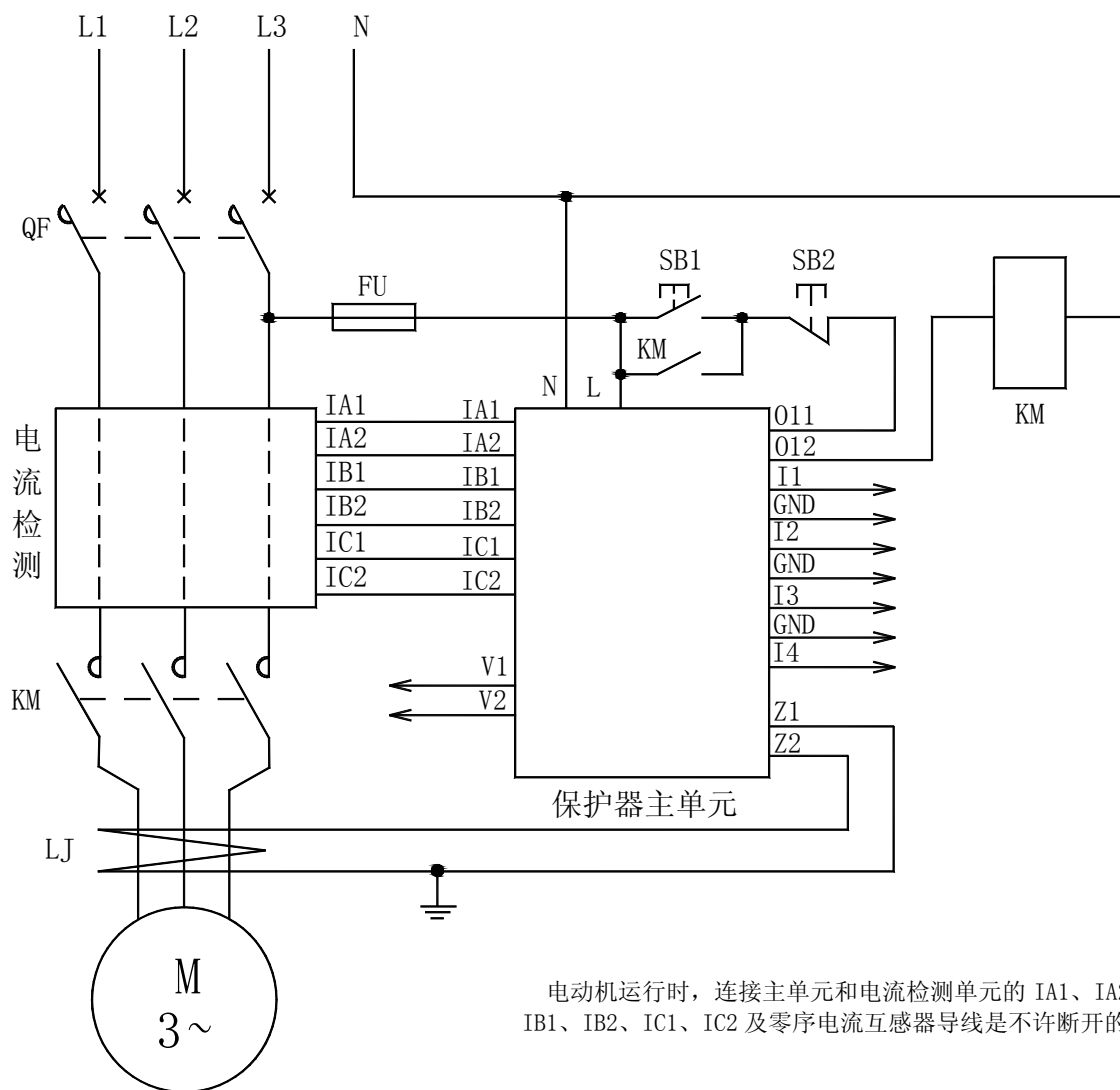
AMDGH-□/D11□ 系列电动机保护器应用电气原理图
