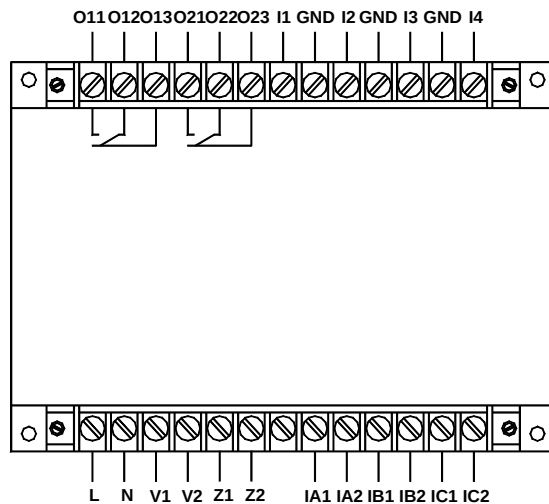
AMDGH-□/D112 系列保护器主单元接线端子图
