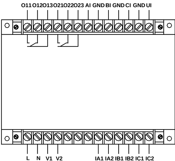
AMDGH-□/D122 系列保护器主单元接线端子图
