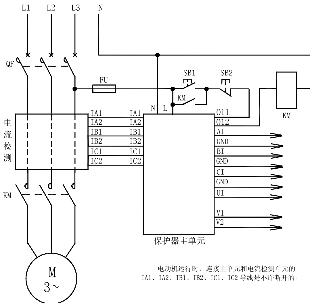
AMDGH-□/D12□ 系列电动机保护器应用电气原理图
