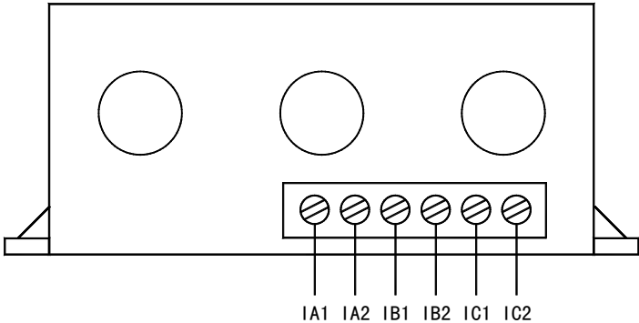
AMDGH-□/D12□ 系列保护器电流检测单元接线端子图
