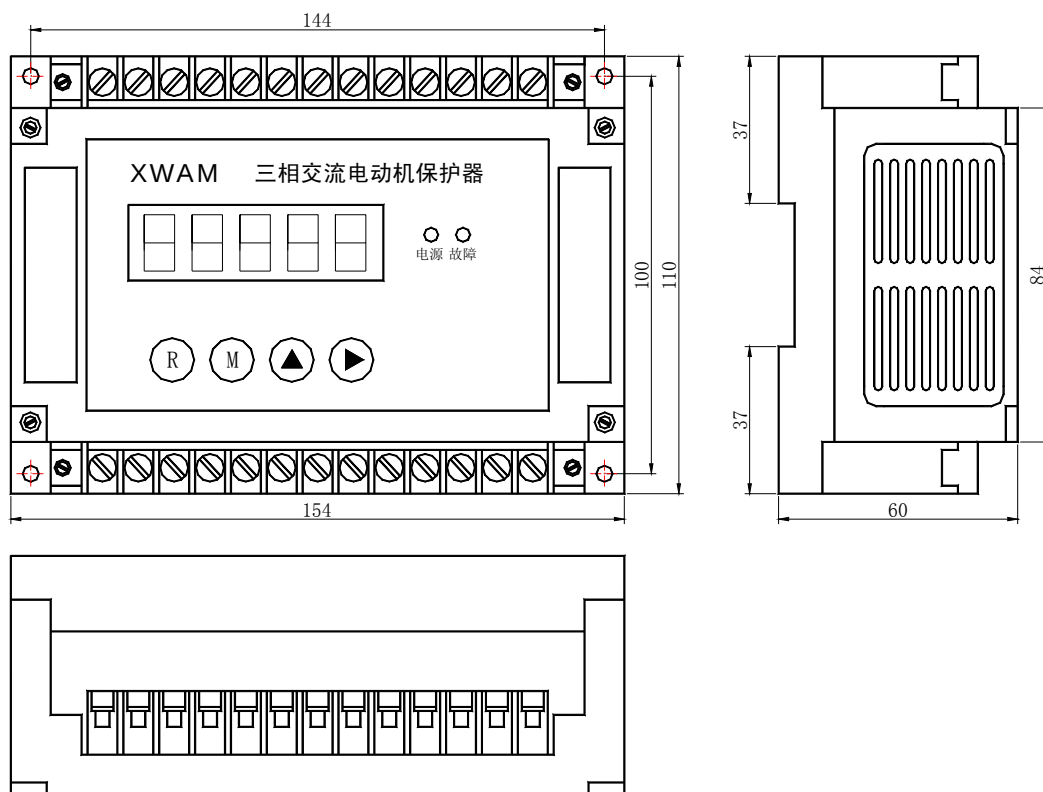
AMDGH-□/D12□ 系列电动机保护器主单元外形及安装孔尺寸
