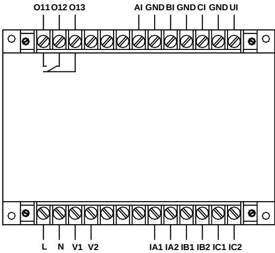
AMDGH-□/D121 系列保护器主单元接线端子图
