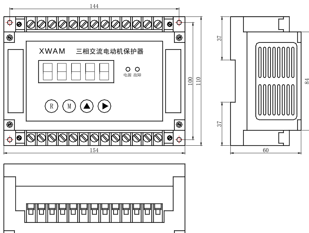
AMDGH-□/D13□ 系列电动机保护器主单元外形及安装孔尺寸
