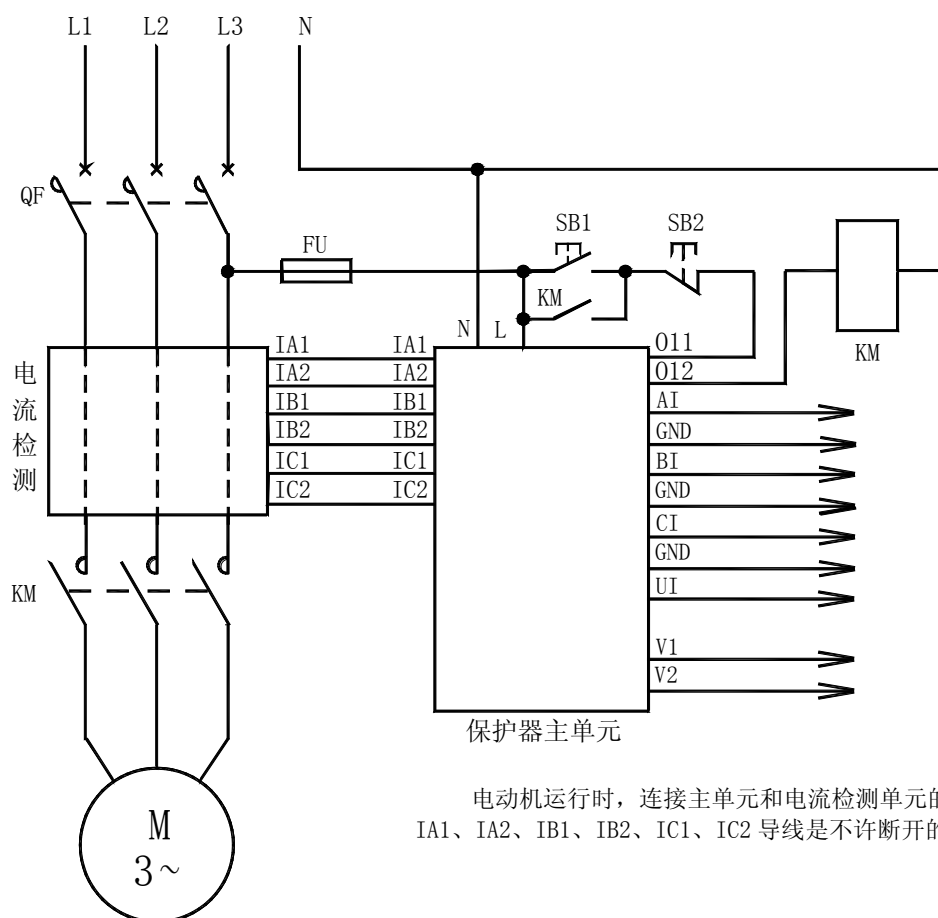
AMDGH-□/D13□ 系列电动机保护器应用电气原理图
