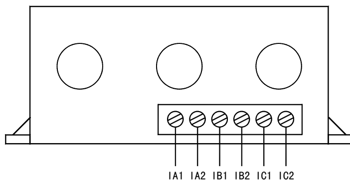
AMDGH-□/D13□ 系列保护器电流检测单元接线端子图
