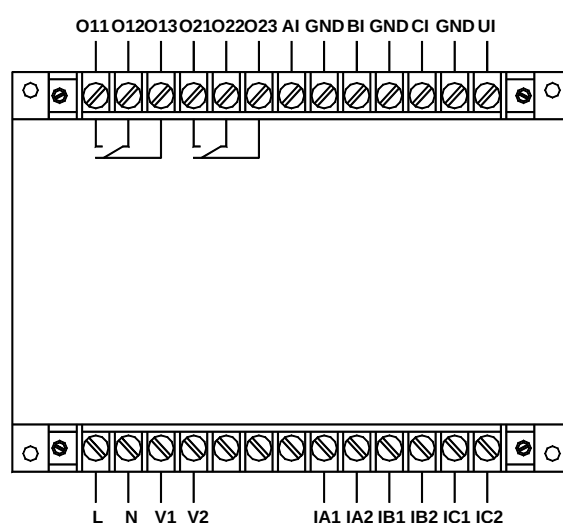
AMDGH-□/□D132 系列保护器主单元接线端子图
