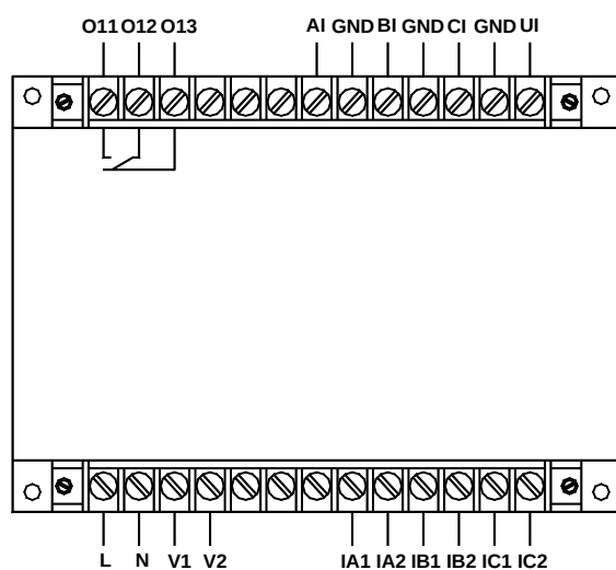
AMDGH-□/□D131 系列保护器主单元接线端子图
