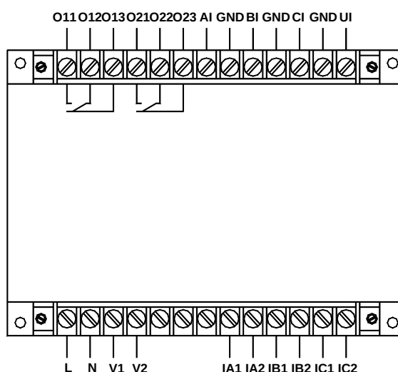
AMDGH-□/D142 系列保护器主单元接线端子图
