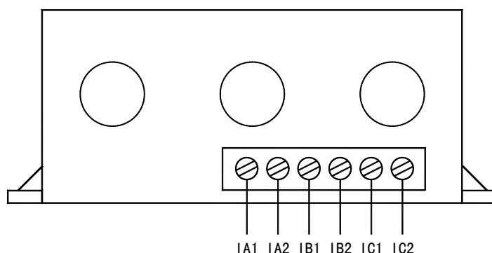
AMDGH-□/□系列保护器电流检测单元接线端子图
