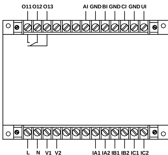
AMDGH-□/D141 系列保护器主单元接线端子图
