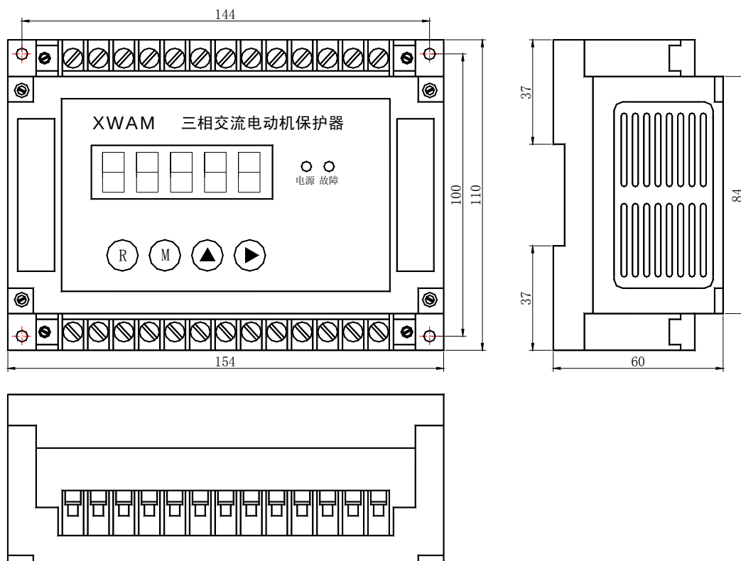
AMDGH-□/D14□ 系列电动机保护器主单元外形及安装孔尺寸
