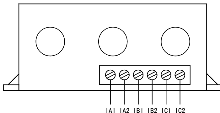
AMDGH-□/□/15□ 系列保护器电流检测单元接线端子图
