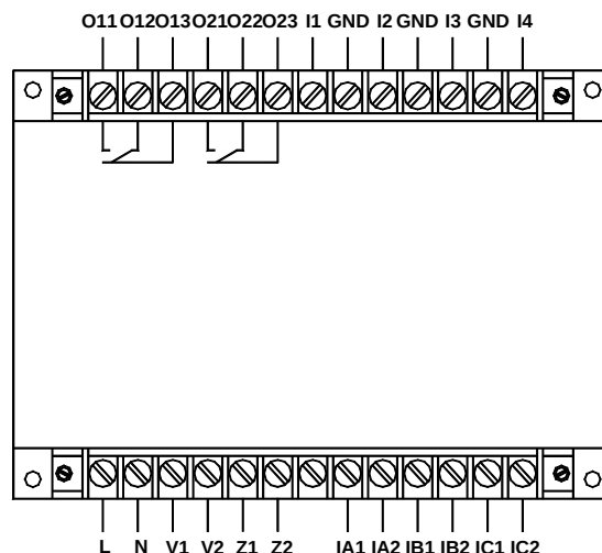
AMDGH-□/□/152 系列保护器主单元接线端子图
