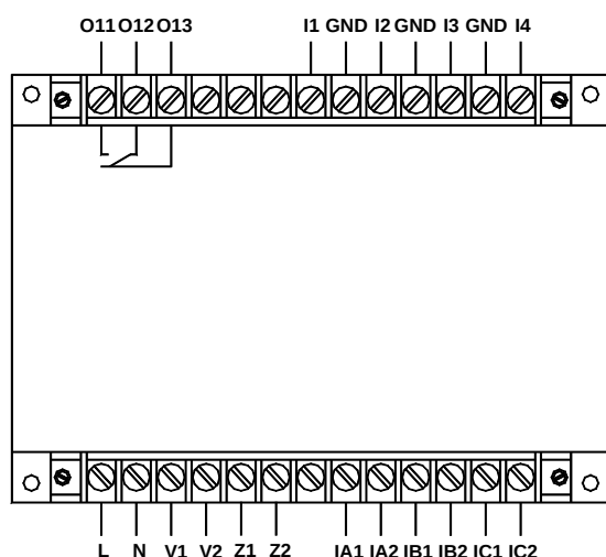
AMDGH-□/□/151 系列保护器主单元接线端子图
