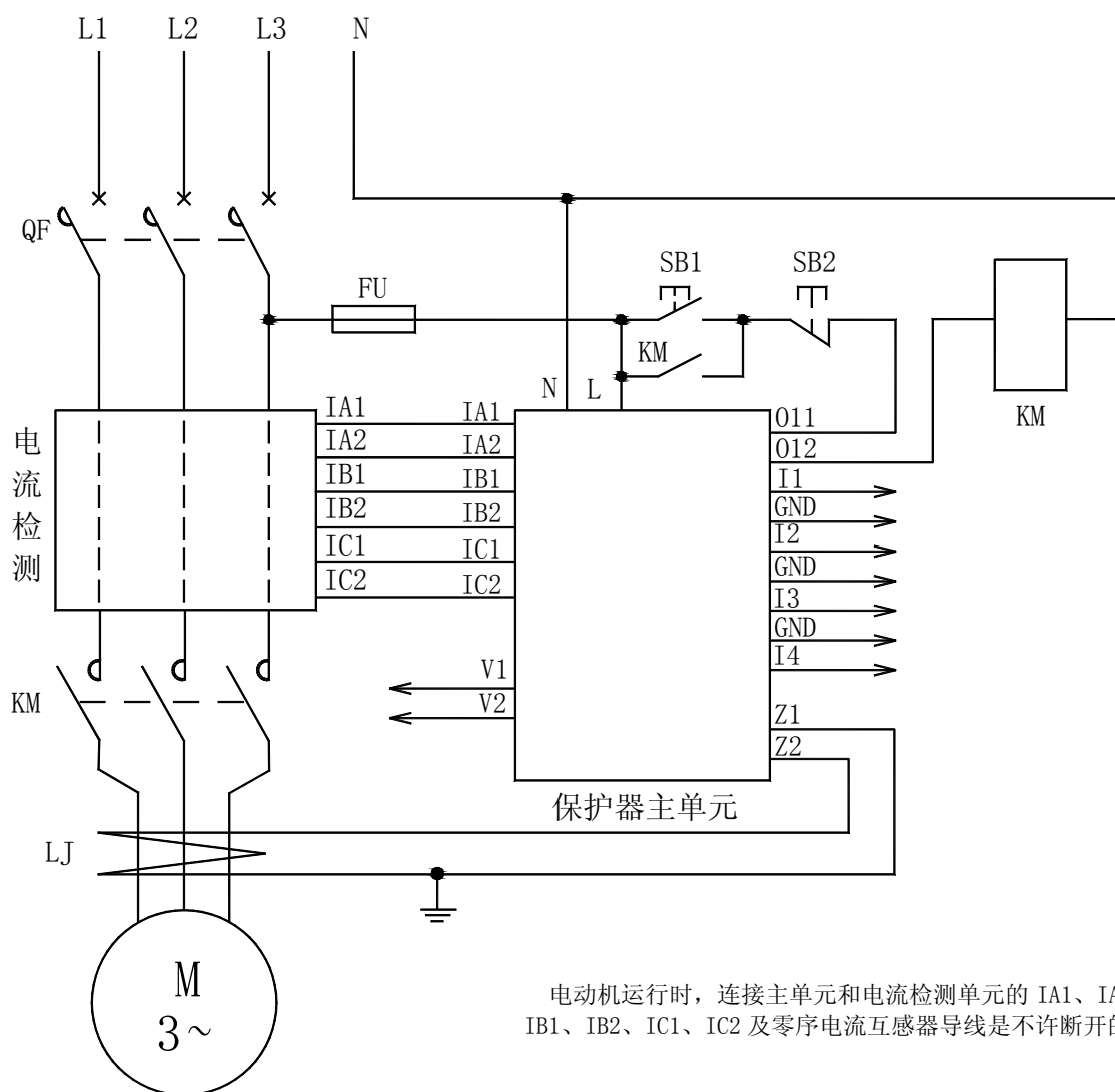
AMDGH-□/D15□ 系列电动机保护器应用电气原理图
