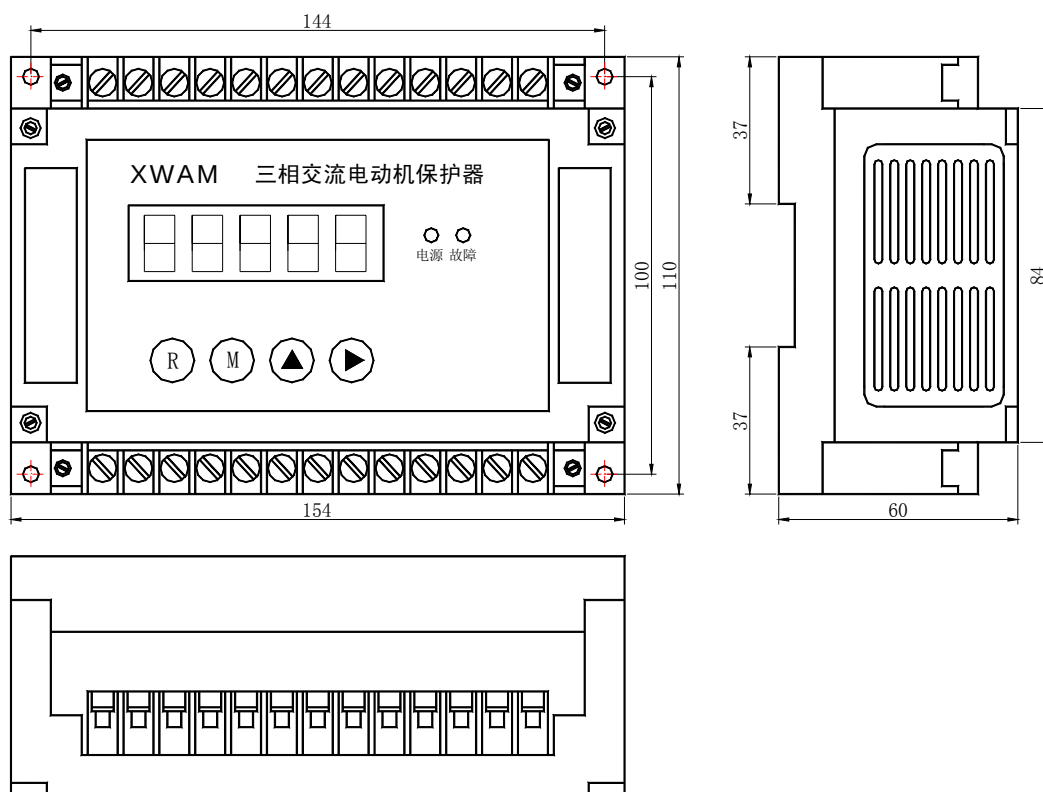
AMDGH-□/□/15□ 系列电动机保护器主单元外形及安装孔尺寸
