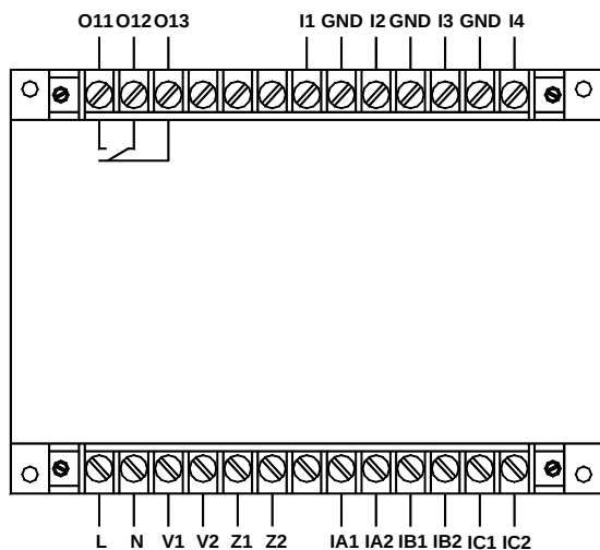
AMDGH-□/D171 系列保护器主单元接线端子图
