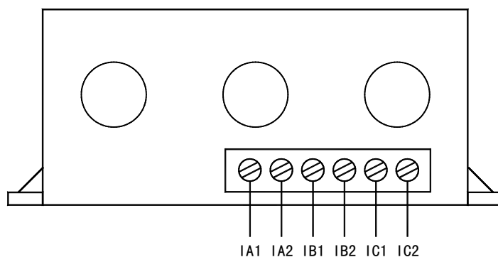
AMDGH-□/D17□ 系列保护器电流检测单元接线端子图
