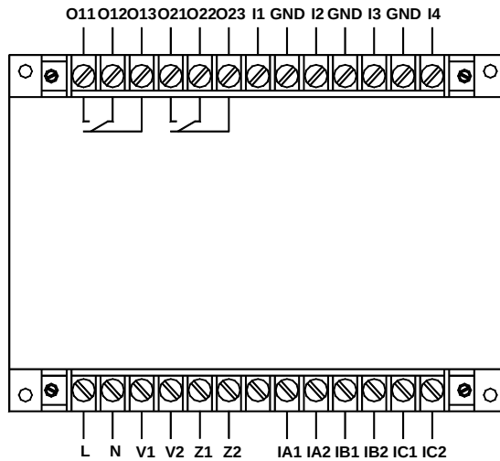
AMDGH-□/D172 系列保护器主单元接线端子图
